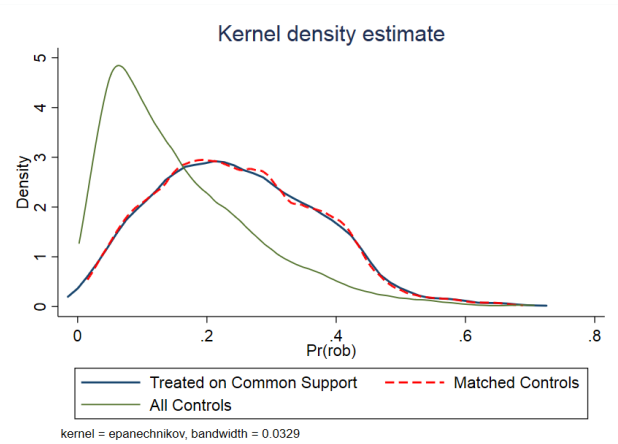
(d) RadiusMatching
