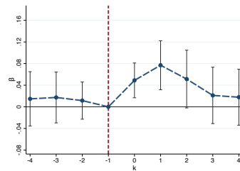
(d) \beta_{rev,P}
