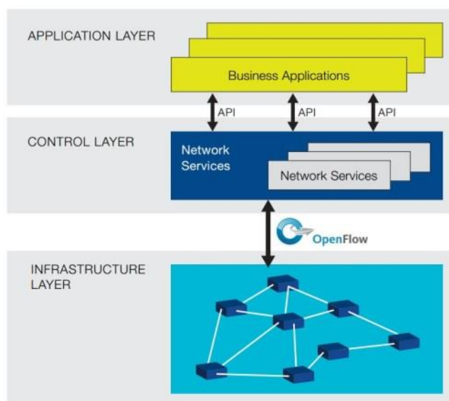
Abbildung 2-1: SDN Netzarchitektur
