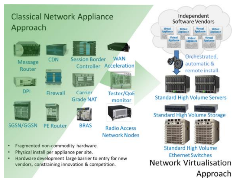
Abbildung 2-4: NFV Ansatz von ETSI
