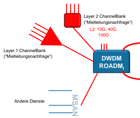
Abbildung 3-5: Übergang der Dienste auf den Ring zur nächsthöheren Netzebene
