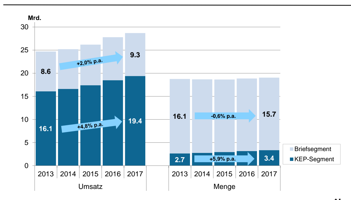
Abbildung 1 Mengen- und Umsatzentwicklung im deutschen Postmarkt (2013-2017)
