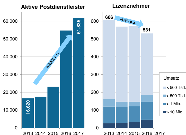
Abbildung 2 Anzahl der Unternehmen im deutschen Postmarkt (2013-2017)
