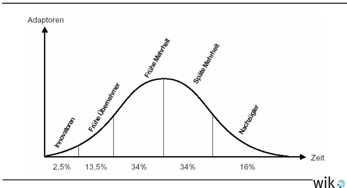
Abbildung 3-3: Die verschiedenen Phasen eines Diffusionsprozesses
