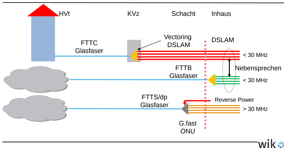
Abbildung 8-1: G.fast, FTTB und VDSL Vectoring, Infrastrukturvergleich
