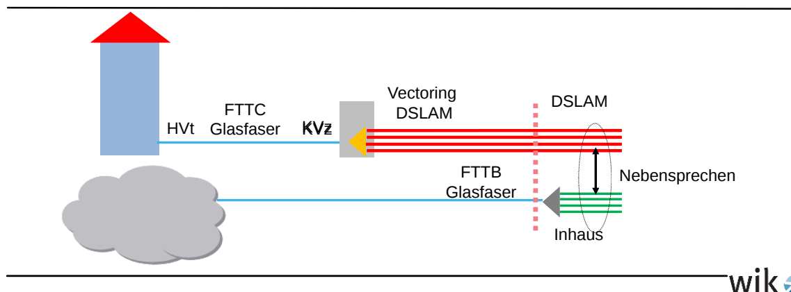
Abbildung 5-1: Koexistenz von FTTC und FTTB
