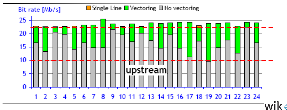
Abbildung 2-6: VDSL Vectoring, Upstream Bandbreiten (Labormessungen Swisscom (s.o.))
