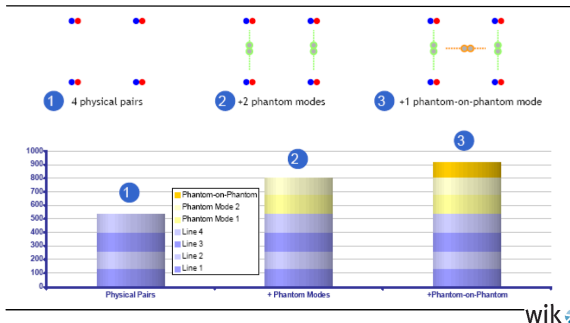
Abbildung 4-1: Bandbreitengewinn aus Phantoming mit 4 DA Bonding und Vectoring bei 400 m Subloop (Bellabs Labordemo)
