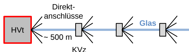
Abbildung 2-11: Kaskadierte VDSL Vectoring DSLAMs
