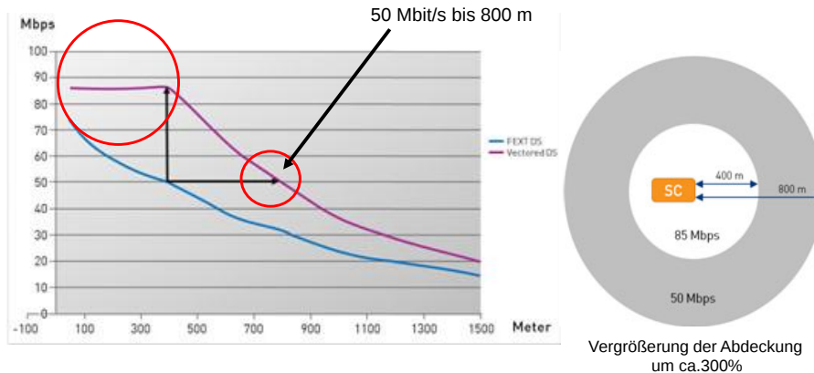
Abbildung 2-7: Reichweitenverbesserung und Vergrößerung der Flächenabdeckung durch VDSL Vectoring
