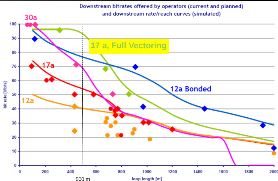
Abbildung 2-4: Bandbreiten - Längen Relationen bei Verbesserungen in VDSL (Simulationen und existierende und geplante Angebote 13 )
