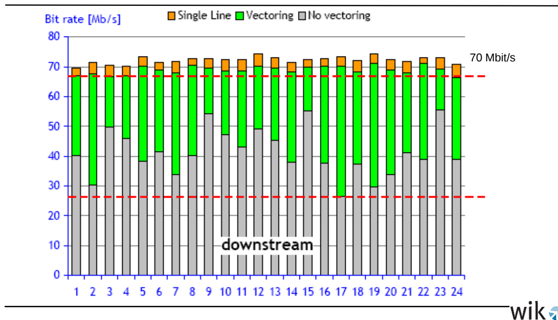
Abbildung 2-5: VDSL Vectoring, Downstream Bandbreiten (Labormessungen Swisscom 14 )
