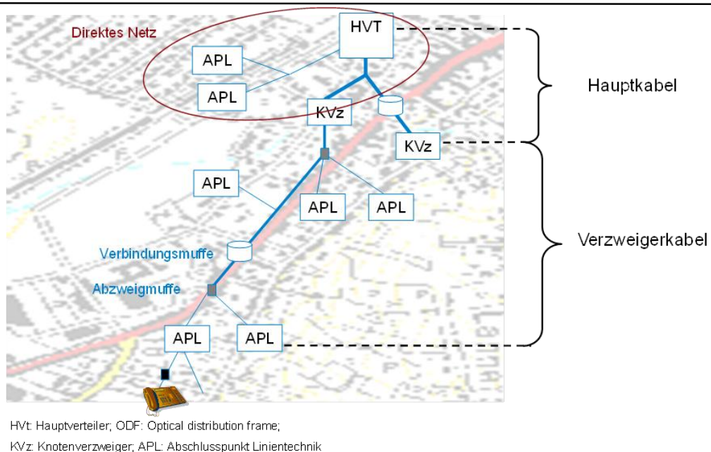
Abbildung 1-1: Prinzip eines Kupfer basierten Teilnehmeranschlussnetzes
