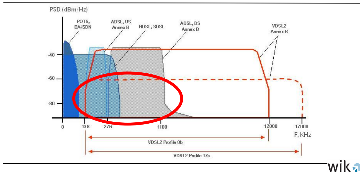
Abbildung 2-9: Frequenzbereiche typischer Signalübertragungen auf einem Teilnehmeranschlusskabel
