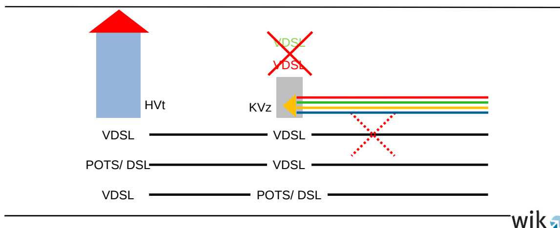
Abbildung 2-10: Kombination von Nutzungen im Anschlussnetz
