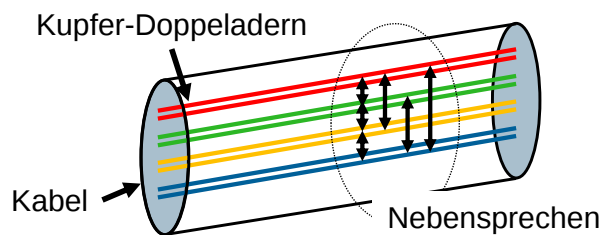
Abbildung 2-2: Nebensprechen
