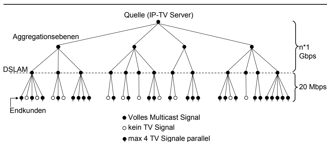
Abbildung 5-2: Schematische Darstellung eines Multicast Baumes
