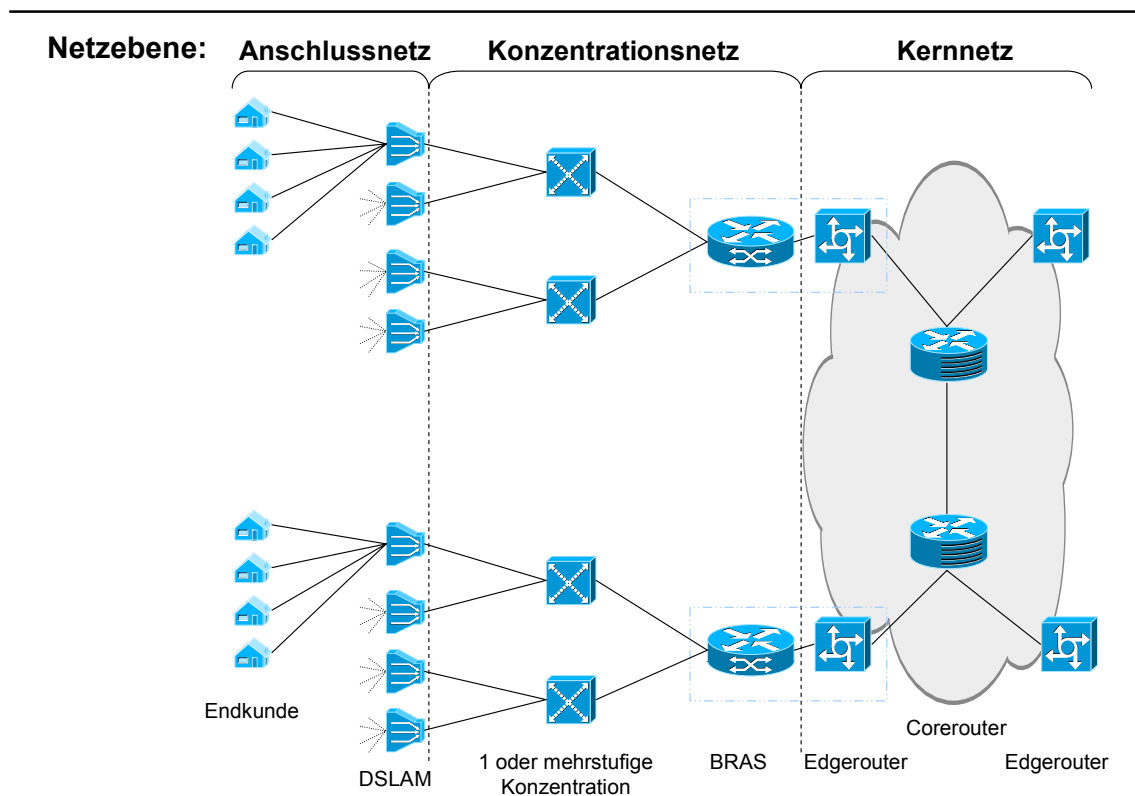
Abbildung 4-1: Netzebenen des Breitbandnetzes
