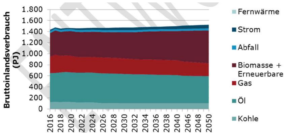
Abbildung 6: Projektion des Primärenergieverbrauchs in Petajoule (Referenzszenario) und des Primärenergiemix von Österreich (Quelle: NEKP 2018:99) 14
