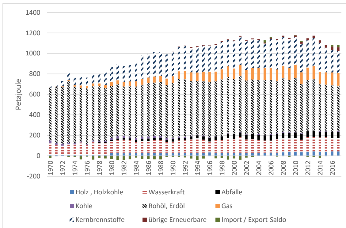
Abbildung 9: Bruttonprimärenergieverbrauch der Schweiz in Petajoule (Quelle: BFS 2018)
