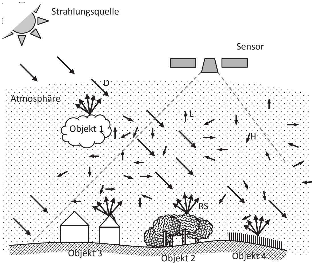
Abbildung 1: Wechselwirkungen Strahlungsquelle - Atmosphäre - Objekt - Sensor (D: Direkte Sonnenstrahlung, H: Himmelsstrahlung, L: Luftlicht, RS: Reflexion und Streuung)
