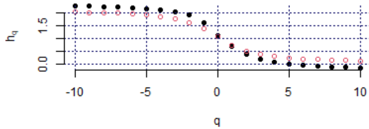
Hurst exponent (USA_NYSE, c2)
