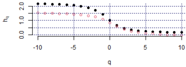
Hurst exponent (GBR_FTSE, c2)
