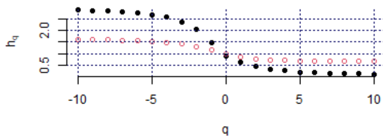
Hurst exponent (JPN_NIKKEI, c1)
