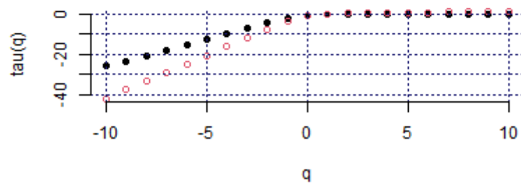
Mass exponent (ZAF_JALSH, c2)
