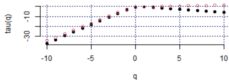
Mass exponent (AUT_ATX, c2)
