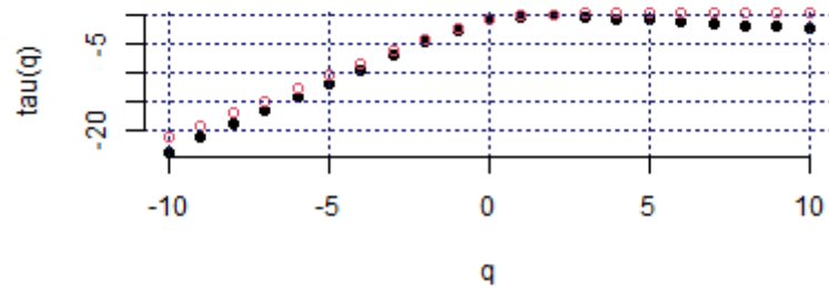
Mass exponent (USA_NYSE, c2)
