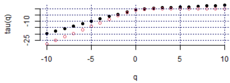
Mass exponent (KOR_KOSPI, c1)
