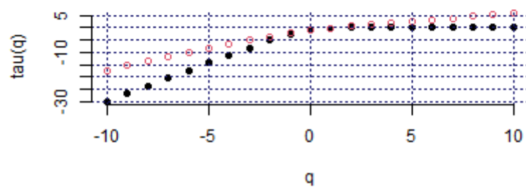
Mass exponent (JPN_NIKKEI, c1)
