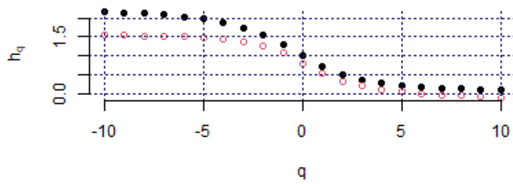
Hurst exponent (KOR_KOSPI, c2)
