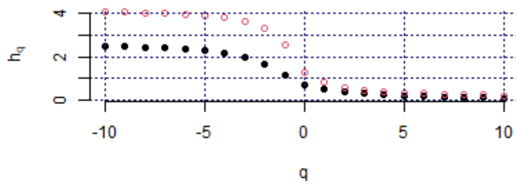
Hurst exponent (ZAF_JALSH, c2)
