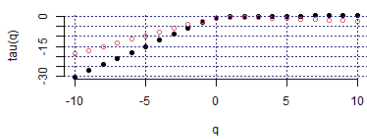
Mass exponent (MEX_SPBMVIPC, c2)
