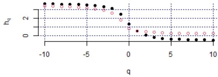
Hurst exponent (AUT_ATX, c2)
