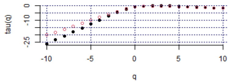
Mass exponent (BRA_IBOVESPA, c2)
