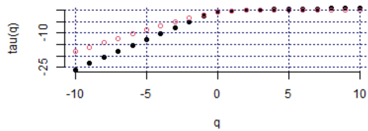
Mass exponent (NZL_NZX, c1)
