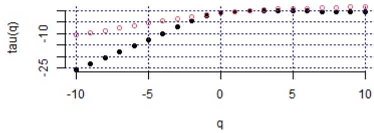
Mass exponent (ZAF_JALSH, c1)
