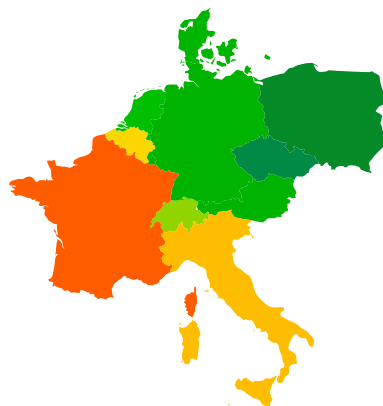
Linear Regression
