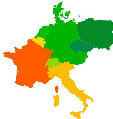
Linear Regression
