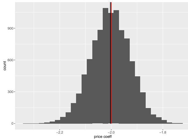
(c) IV-logit “BLP \times N_t ”
