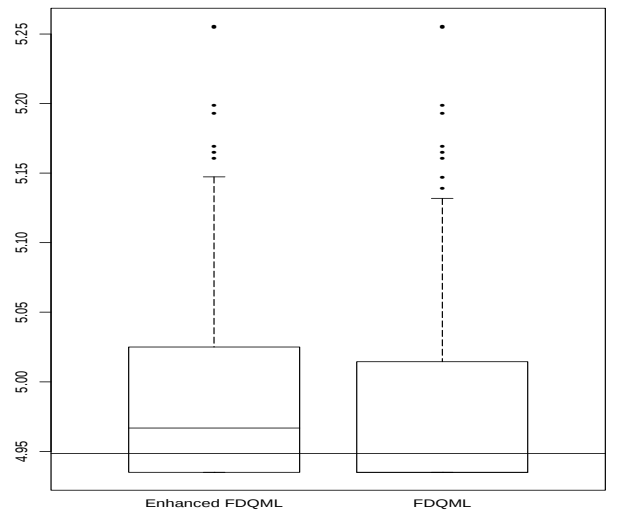
(d) \hat{\sigma}_\epsilon^2 ( \sigma_\epsilon^2 = 4.94847 )
