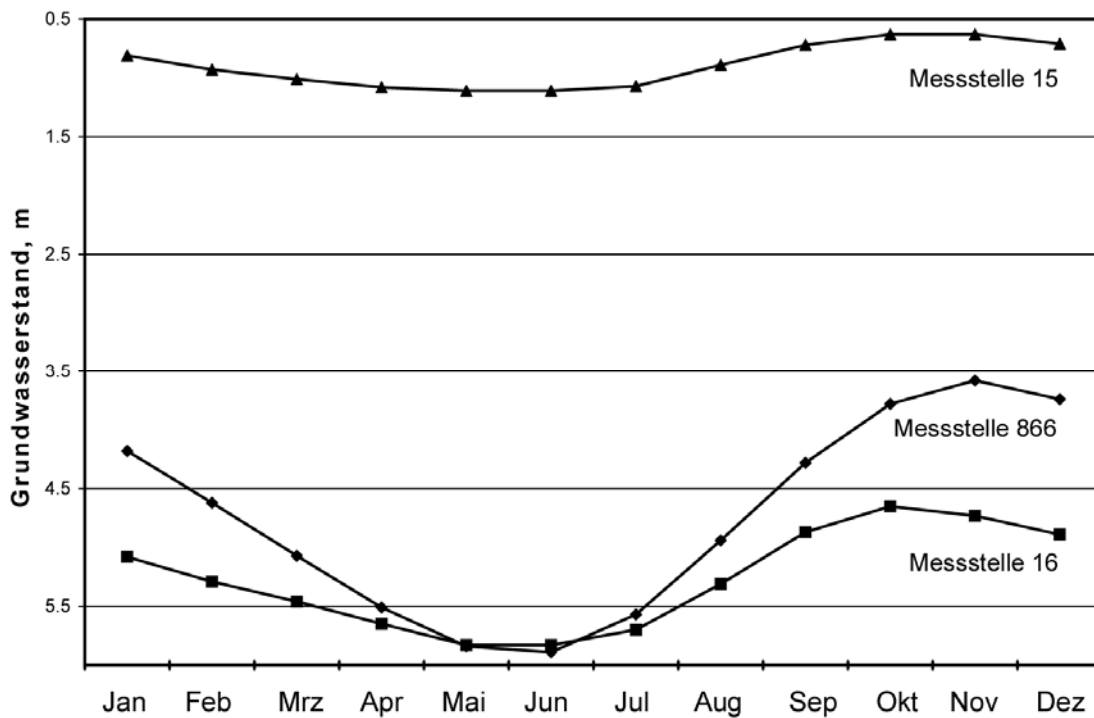
Abb. 24: Jahresgang des Grundwasserspiegels an den Messstellen 866, 16 und 15
