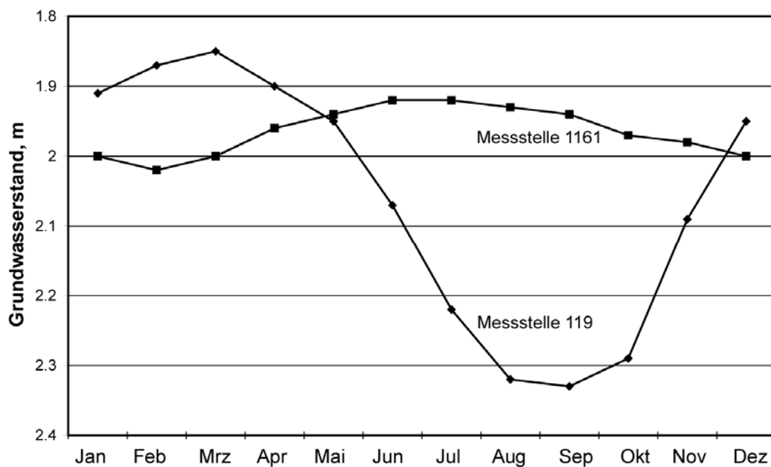
Abb. 25: Jahresgang des Grundwasserspiegels an den Messstellen 119 und 1161
