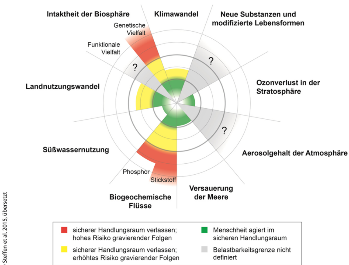
Abbildung 1: Planetare Grenzen
