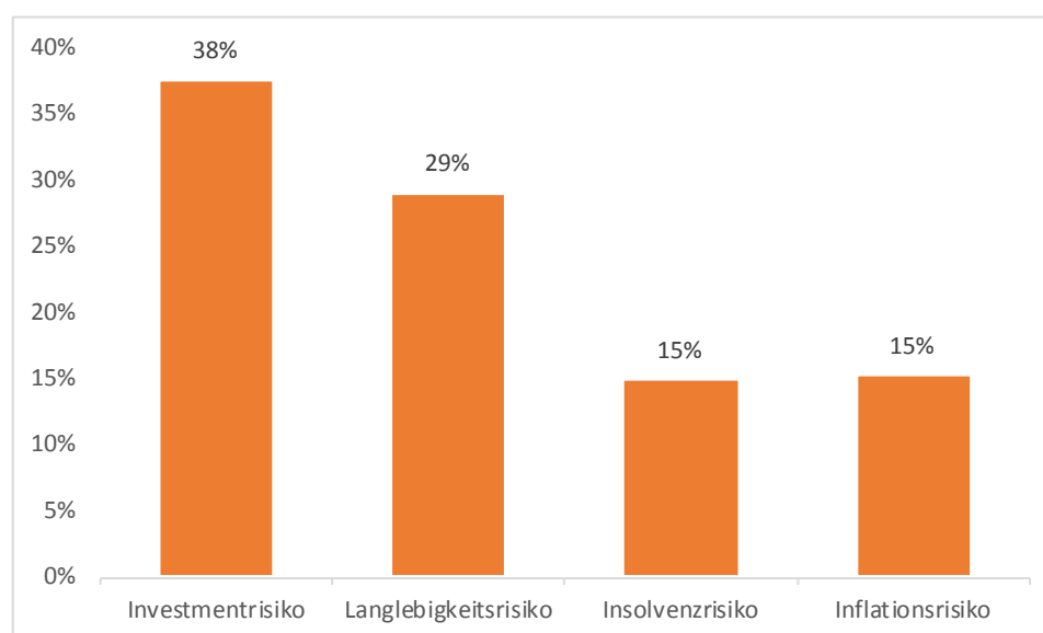
Abbildung 2: BAV-Indikator: Risikoprofil
