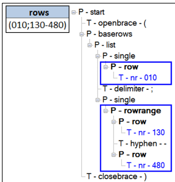
Abbildung 7: Parsebaum der Basiszeilenrestriktion (010;130-480)
