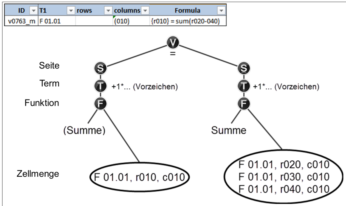
Abbildung 25: Abstrakter Syntaxbaum einer Regel
