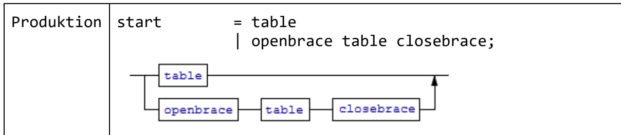
Abbildung 11: Grammatik der Basistabellen
