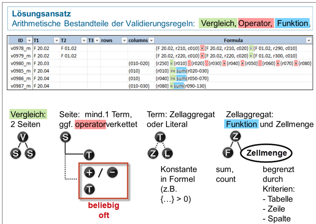
Abbildung 18: Arithmetische Bestandteile von Validierungsregeln
