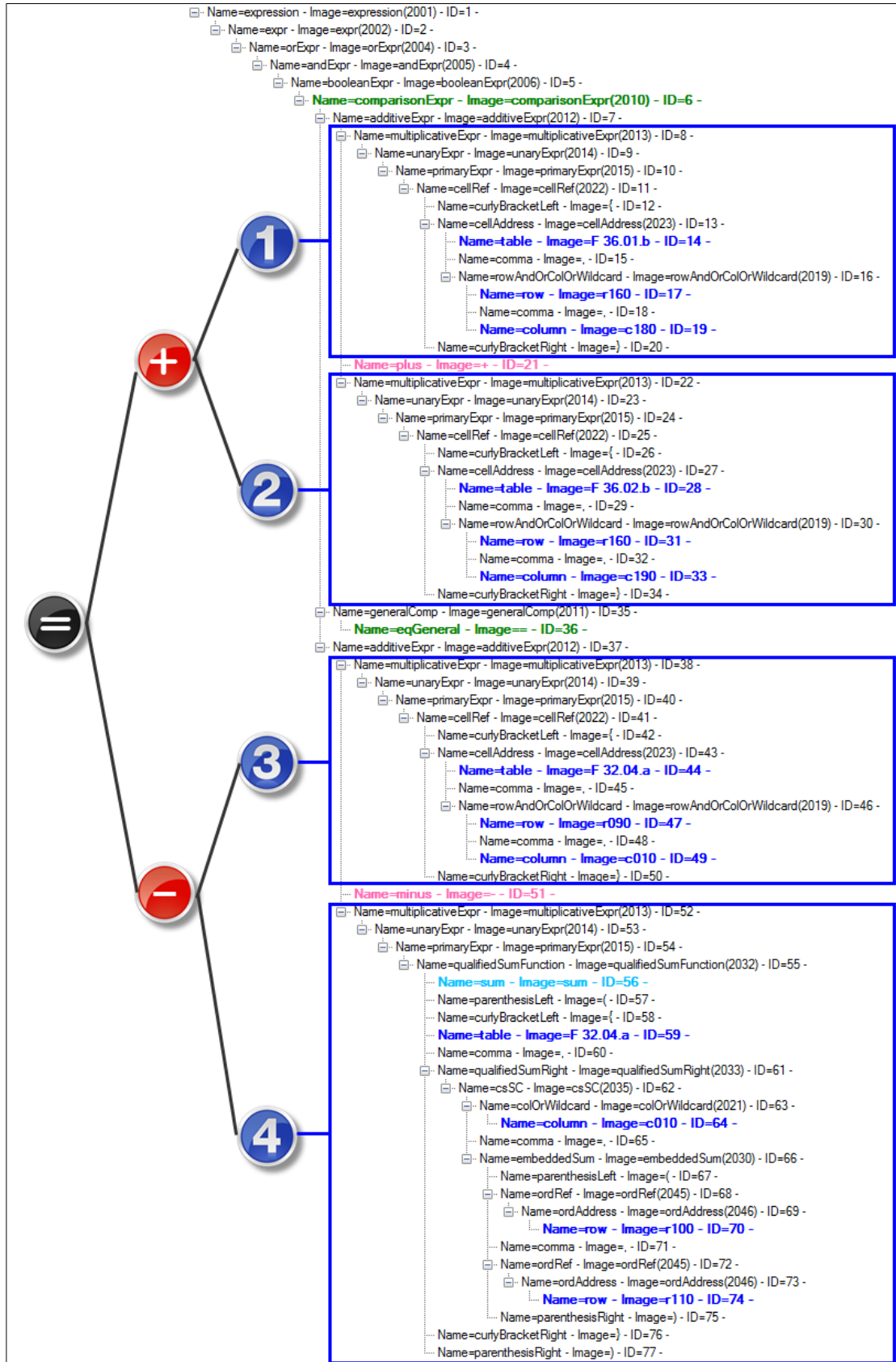
Abbildung 32: Zusammenhang zwischen Parsebaum und AST in Regel v2927_m
