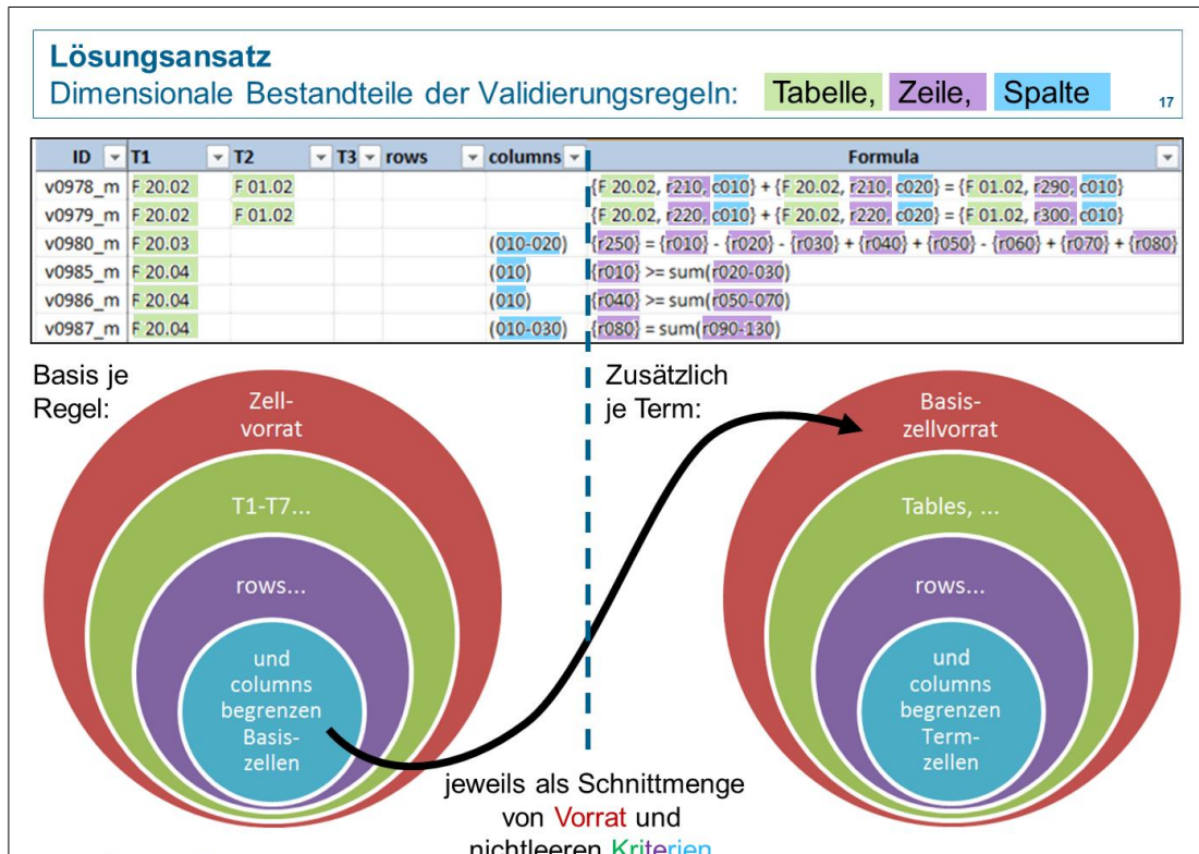
Abbildung 17: Dimensionale Bestandteile von Validierungsregeln
