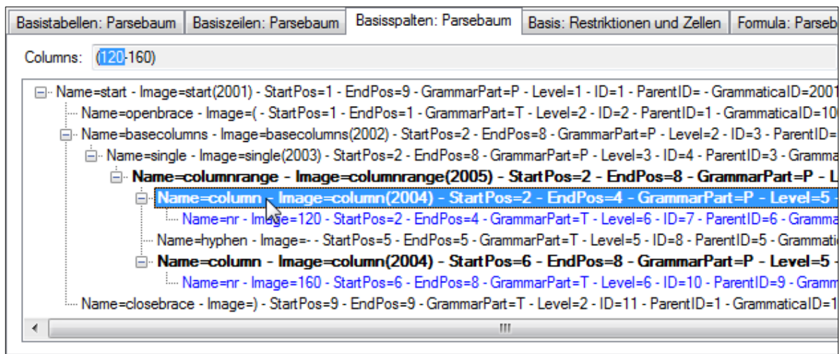
Abbildung 16: Parsebaum eines Basiszeilentextes als TreeView
