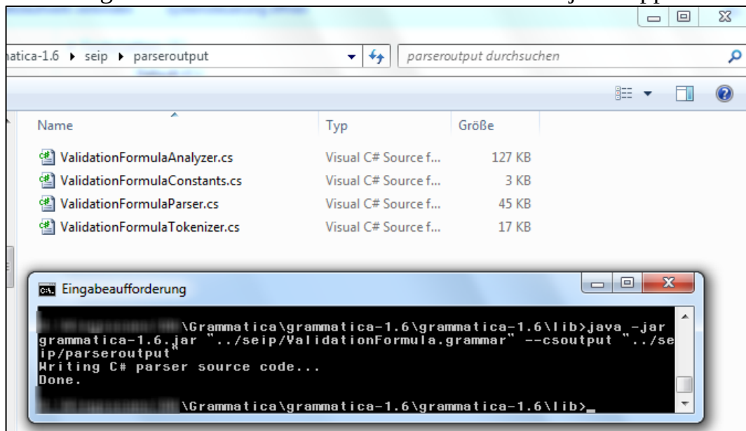
Abbildung 12: Parsergenerierung mit Grammatica
