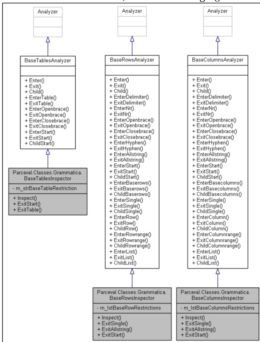
Abbildung 13: Inspector-Klassen der Basisrestriktionen
