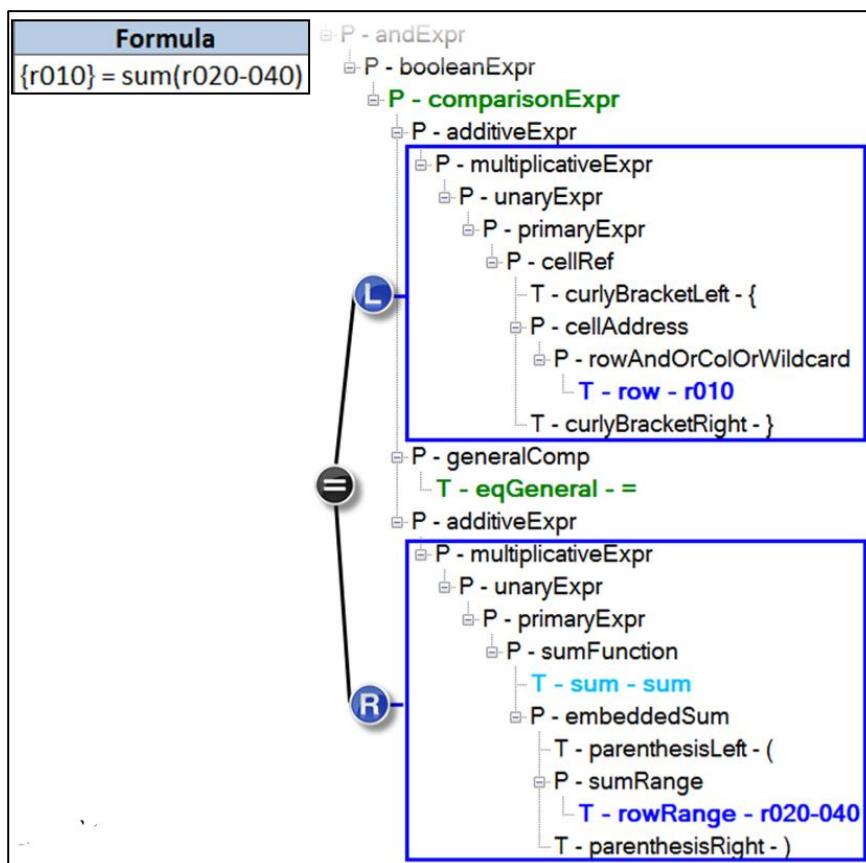
Abbildung 8: Parsebaum einer Formel (Auszug)
