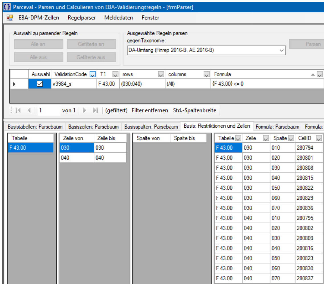
Abbildung 23: Erkannte Basiskriterien und resultierende Basiszellen
