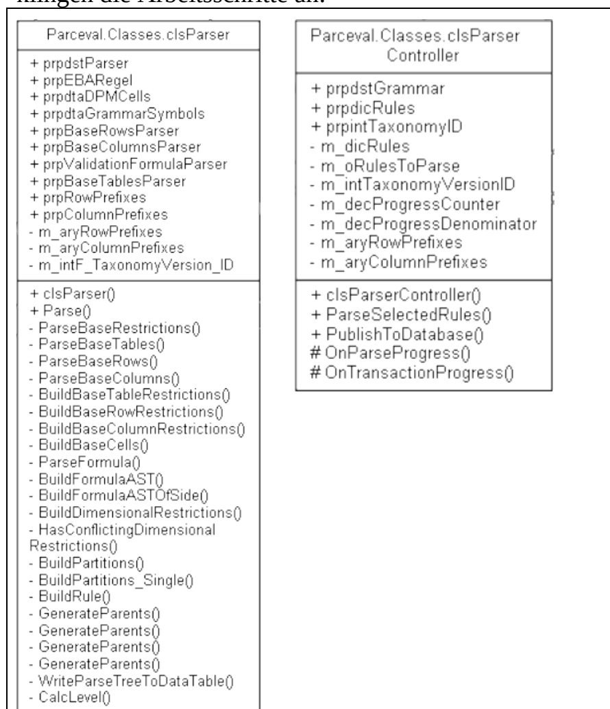
Abbildung 19: UML-Klassendiagramme der Klassen zu Parsersteuerung
