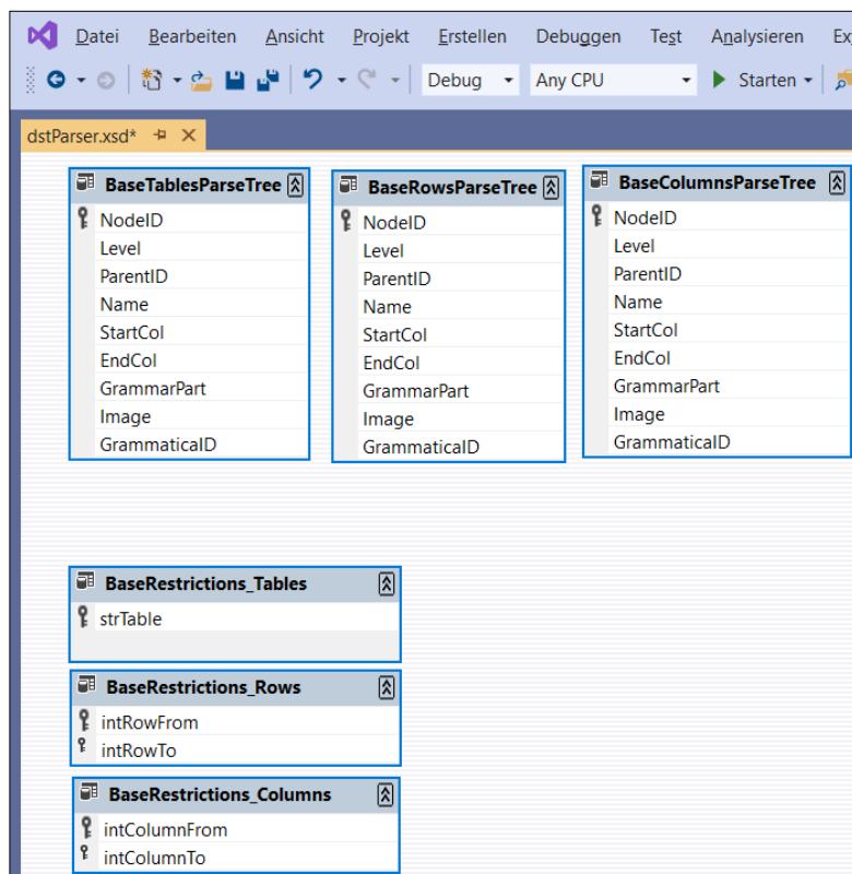
Abbildung 21: DataSet dstParser (Auszug)
