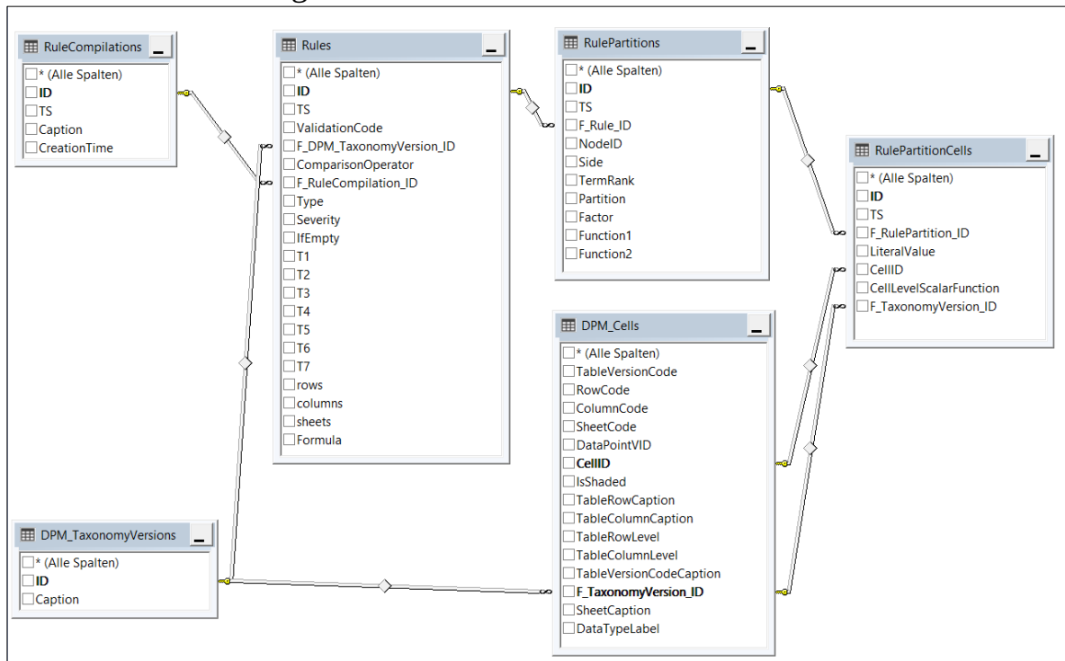
Abbildung 28: Teildatenmodell für die ASTs der EBA-Validierungsregeln
