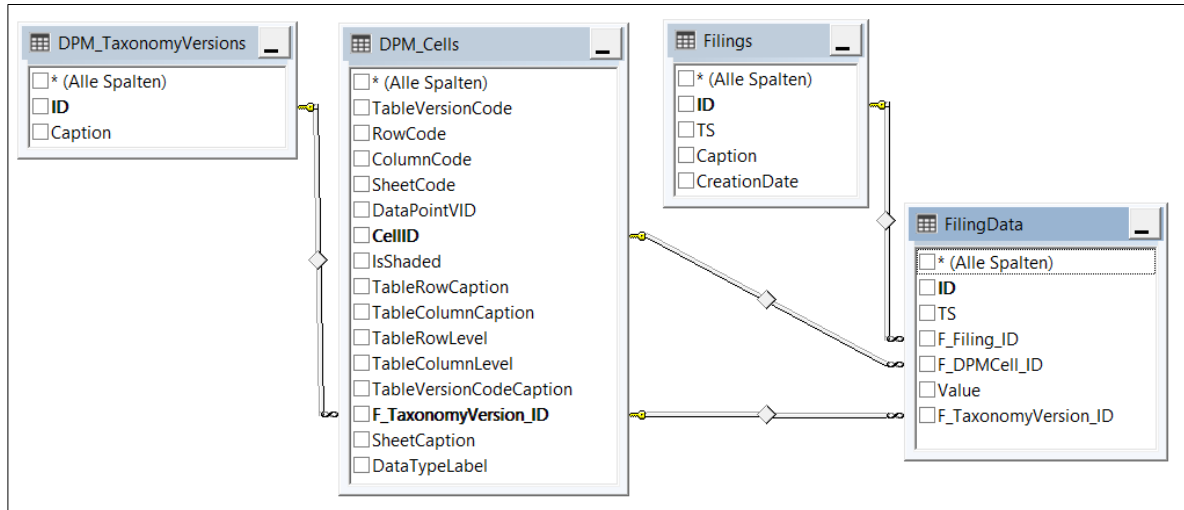
Abbildung 35: Teildatenmodell der Meldedaten
