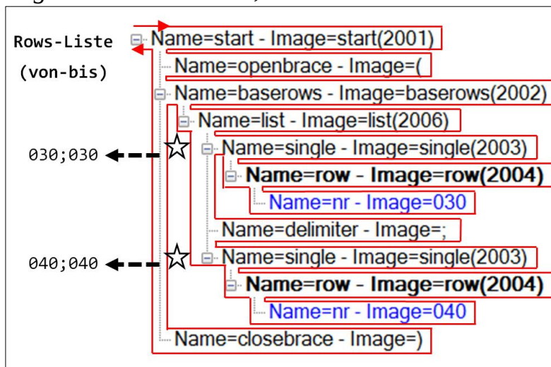
Abbildung 22: tree walk des Parsebaums der Basiszeilenrestriktion (030;040)
