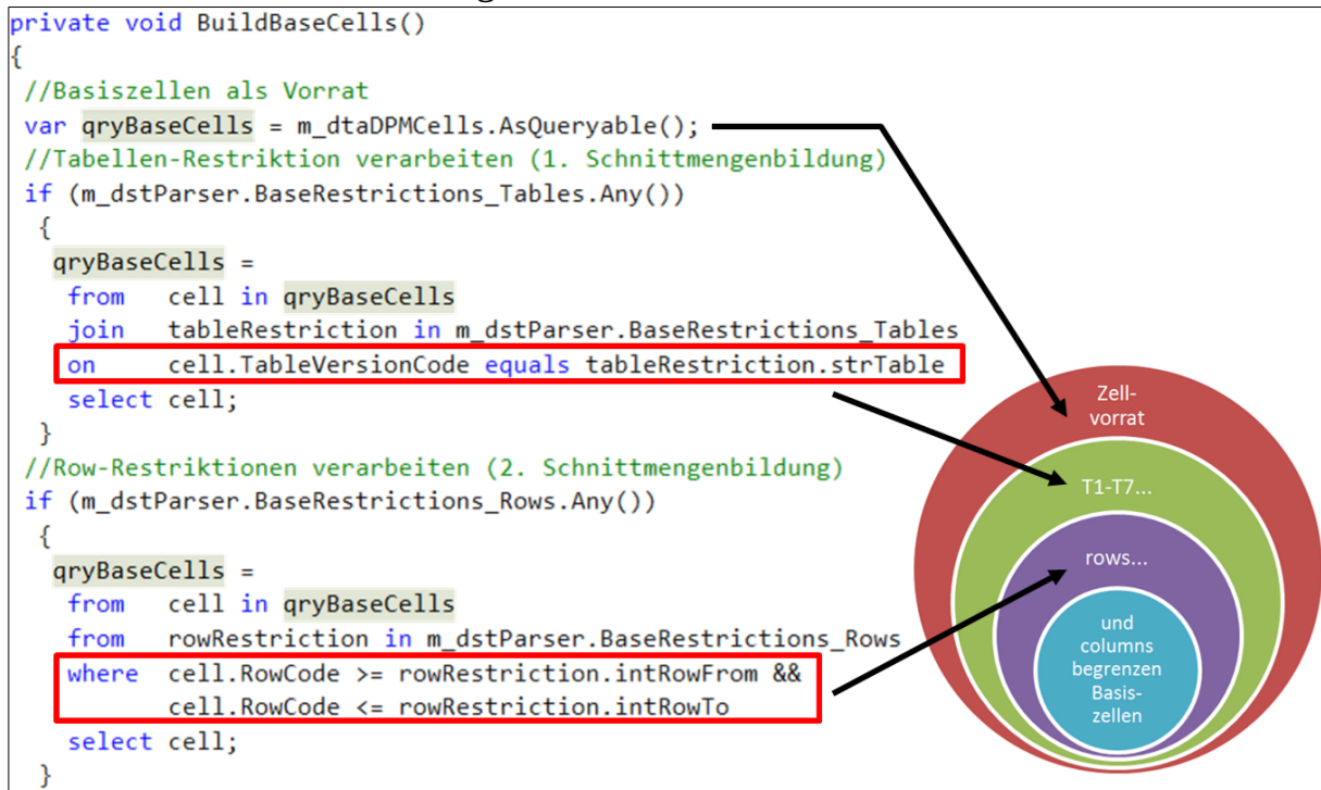
Abbildung 24: Sequenzielle Schnittmenge der Basiskriterien (Auszug)
