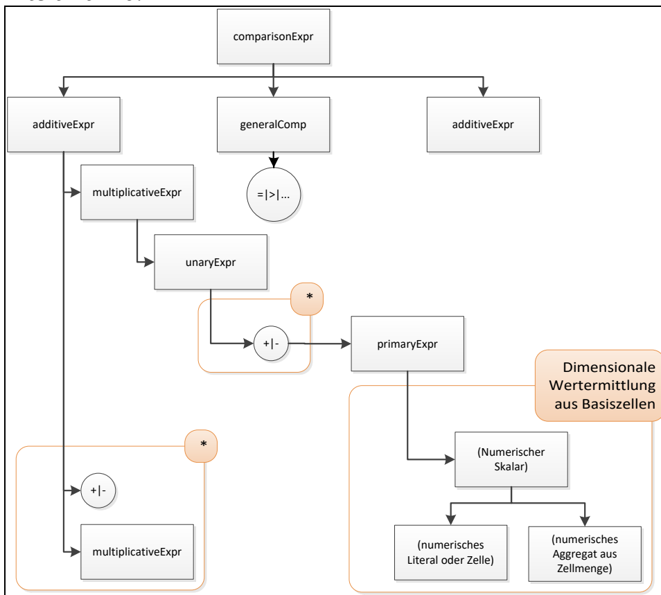
Abbildung 27: Aufbau des abstrakten Syntaxbaums der Formel (Regelskelett)
