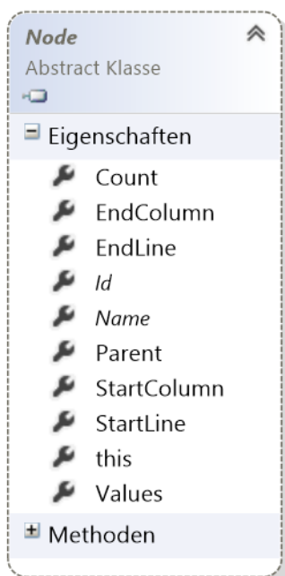
Abbildung 14: Klasse Node
