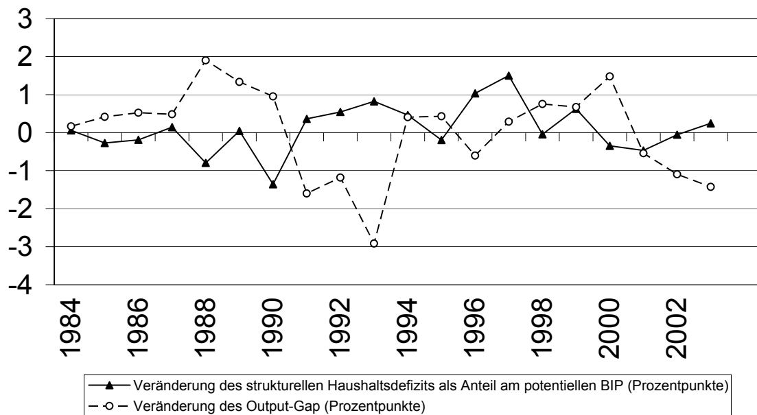
Abb. 9: Veränderung des strukturellen Budgetsaldos und des Output-Gaps in den USA, 1984-2003
