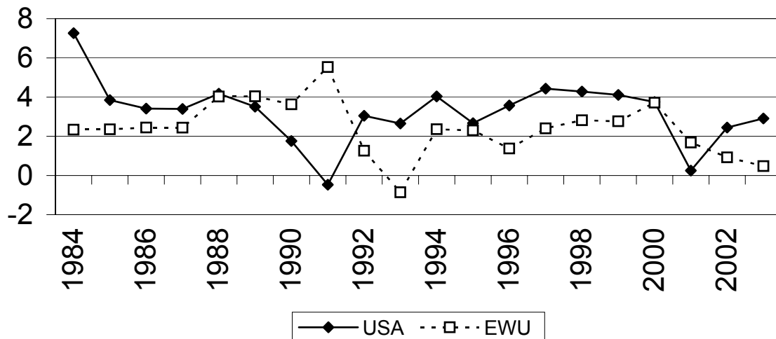
Abb. 1: Wachstumsrate des realen BIP in der EWU und den USA, 1984 - 2003, in % Quelle: OECD (2003)
