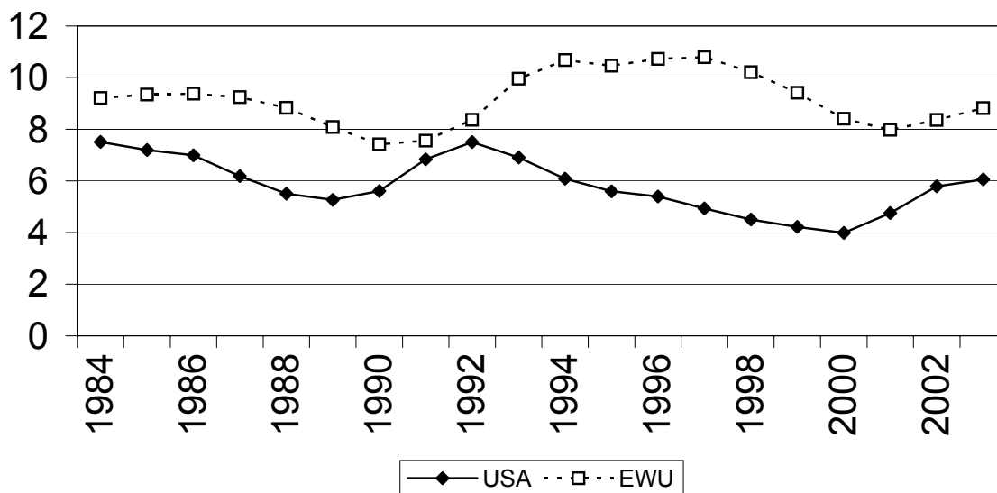
Abb. 2: Arbeitslosenquote in der EWU und den USA, 1984-2003, in % Quelle: OECD (2003)
