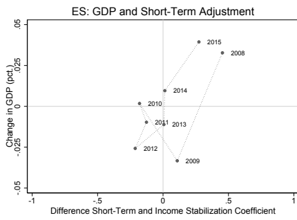
(c) ES
