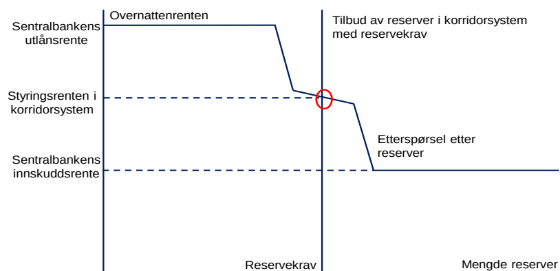
Figur 3.2. Etterspørsel etter og tilbud av sentralbankreserver i et korridorsystem med reservekrav
