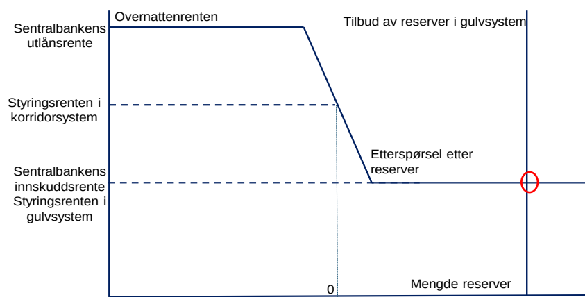
Figur 3.3. Etterspørsel etter og tilbud av sentralbankreserver i et gulvsystem
