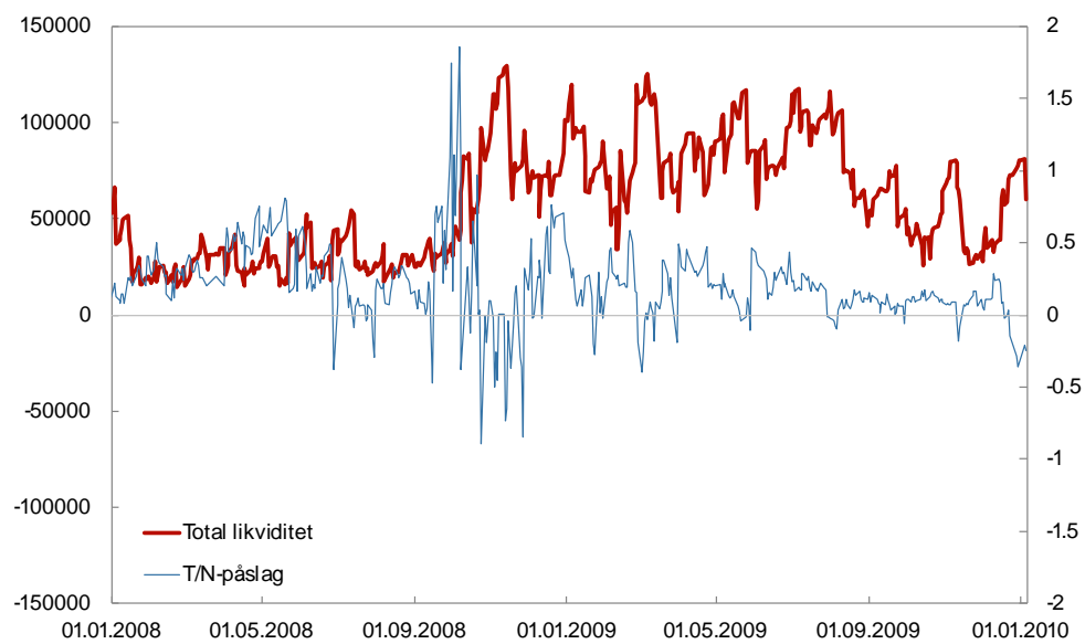
Figur 4: Total likviditet (venstre akse, millioner kroner) og differansen mellom tomorrow-next-renten og forventet styringsrente (høyre akse, basispunkter)
