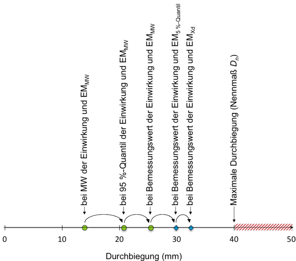
Abbildung 15: Veranschaulichung der Schritte zur Berechnung der Durchbiegung bei Veranschlagung des Bemessungswertes der Einwirkung und dem Biege-Elastizitätsmodul _{Xd} (Bemessungswert der Baustoffeigenschaft) sowie des Nennwertes der maximalen Durchbiegung.
