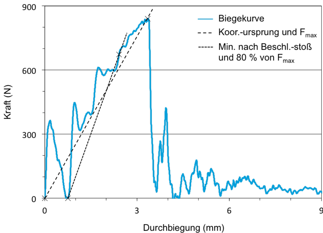
Abbildung 10: Exemplarische Darstellung einer Biegekurve im Kraft-Durchbiegungs-Diagramm mit durch die Punkte „Koordinatenursprung“ und „ F_{max} “ sowie „Kraftminimum zwischen dem Kraftmaximum des Beschleunigungsstoßes und der eigentlichen Biegekurve“ und „80 % von F_{max} “ verlaufenden Geraden, auf Basis deren die Steigung der dynamische Biege-Elastizitätsmodul berechnet wird.
