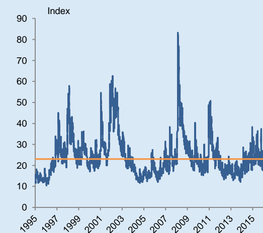
Abbildung 9: VDAX 1995–2016
