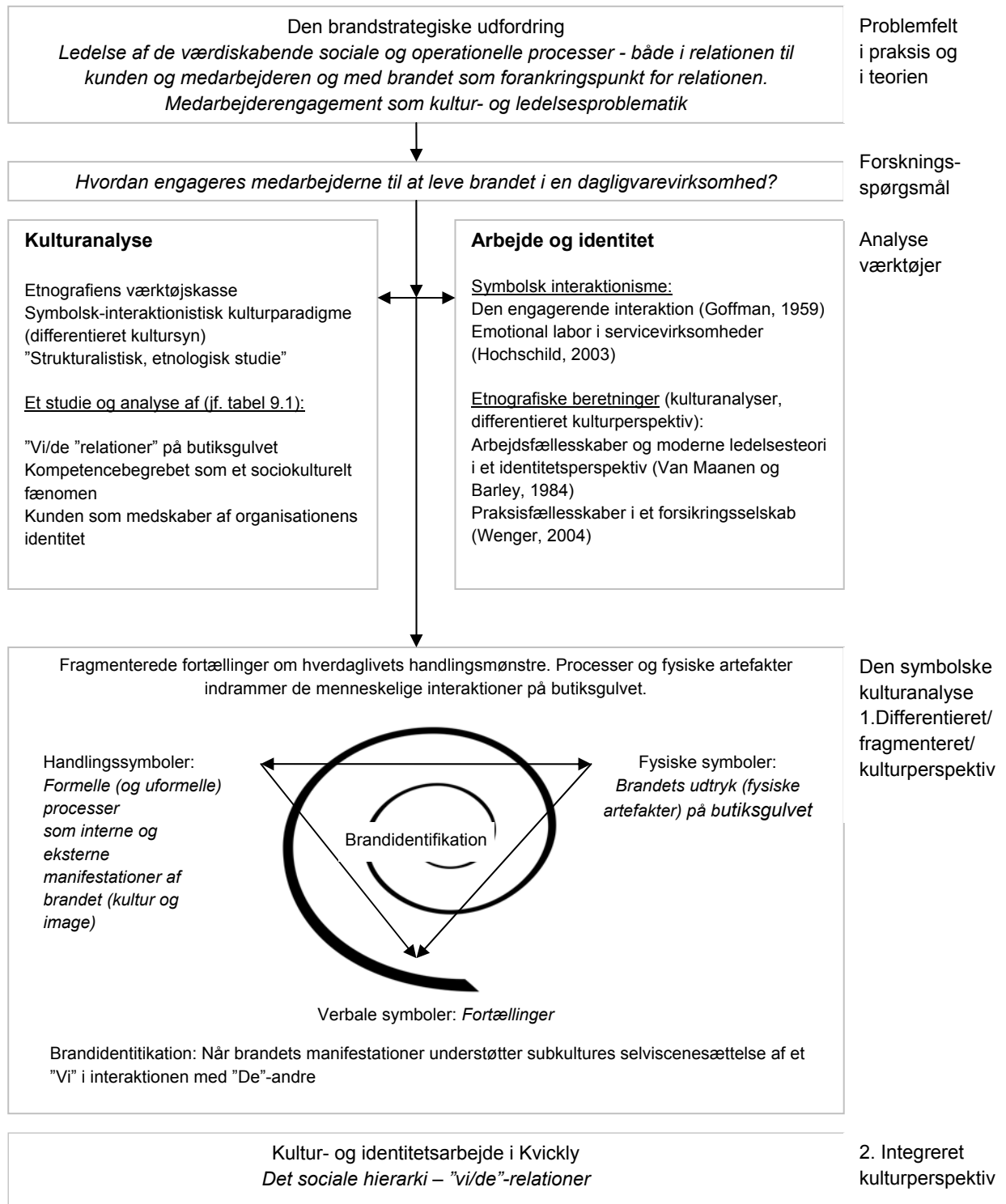
Figur 10.3 Analysens struktur
