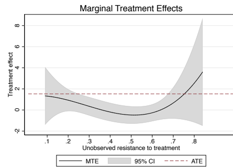
(d) Polynomial Degree 3
