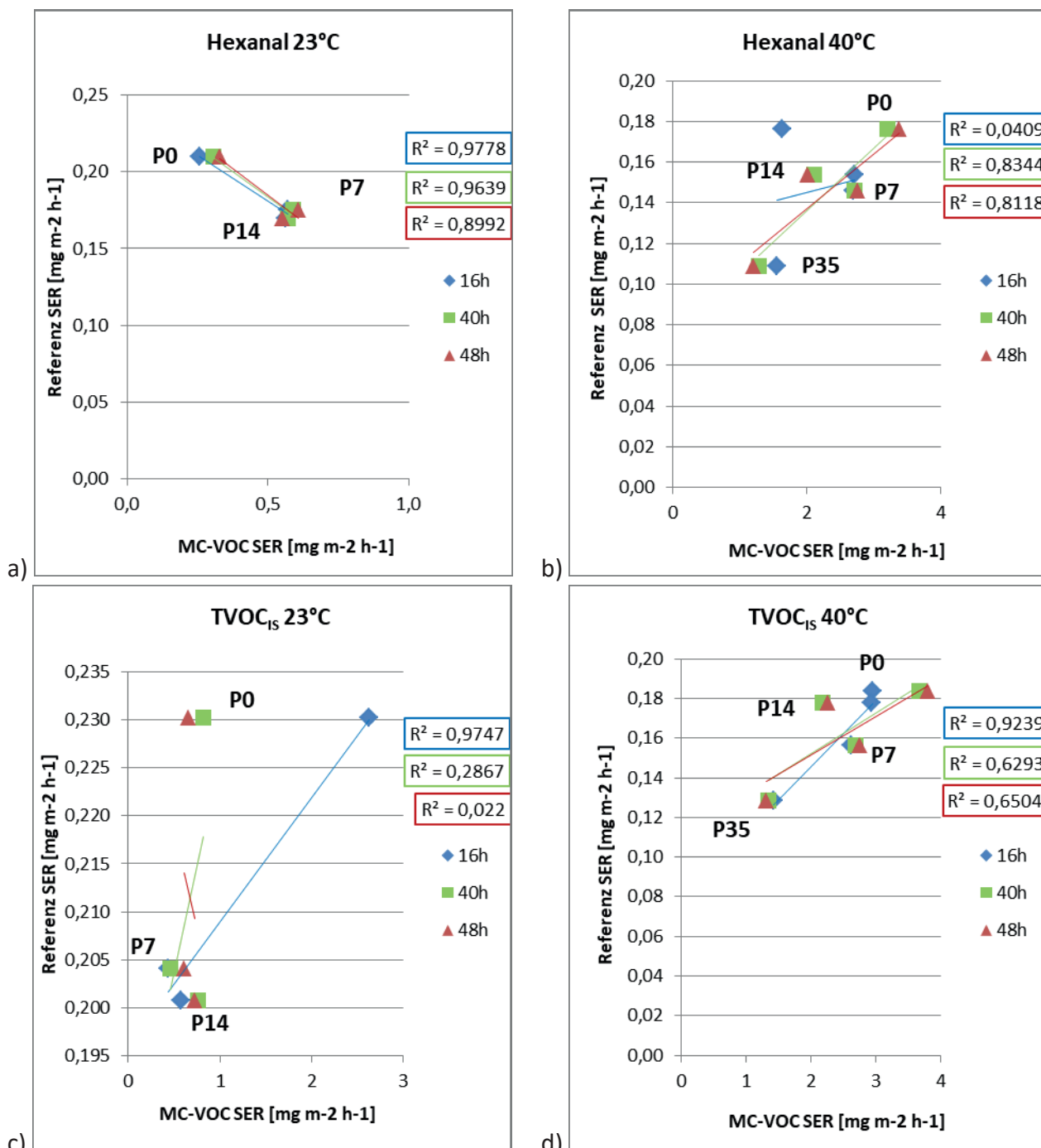
Abbildung 21: Korrelationen für Hexanal (a, b) und TVOC 15 (c, d) zwischen MC-VOC und Referenztest aus Ergebnissen von nicht klimatisierter und klimatisierter Pappel-OSB bei variierender Konditionierungsdauer und Prüftemperatur
