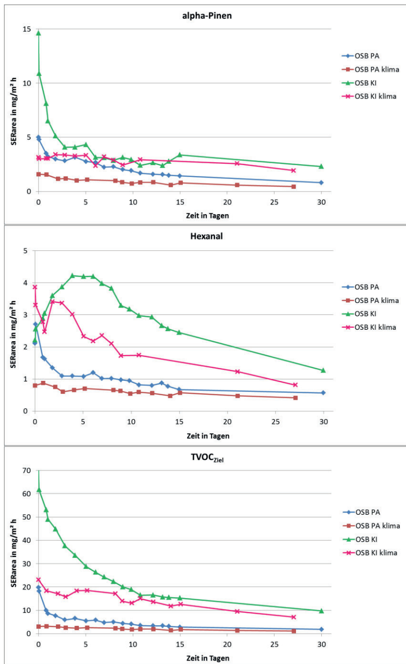
Abbildung 28: Zeitlicher Verlauf der Abgabe von \alpha -Pinen (oben), Hexanal (Mitte) und TVOC Ziel (unten) von unklimatisierten OSB-Proben mit einer Deckschicht aus Pappel (OSB PA ) bzw. Kiefer (OSB KI ) sowie von klimatisierten OSB-Proben mit Deckschicht
