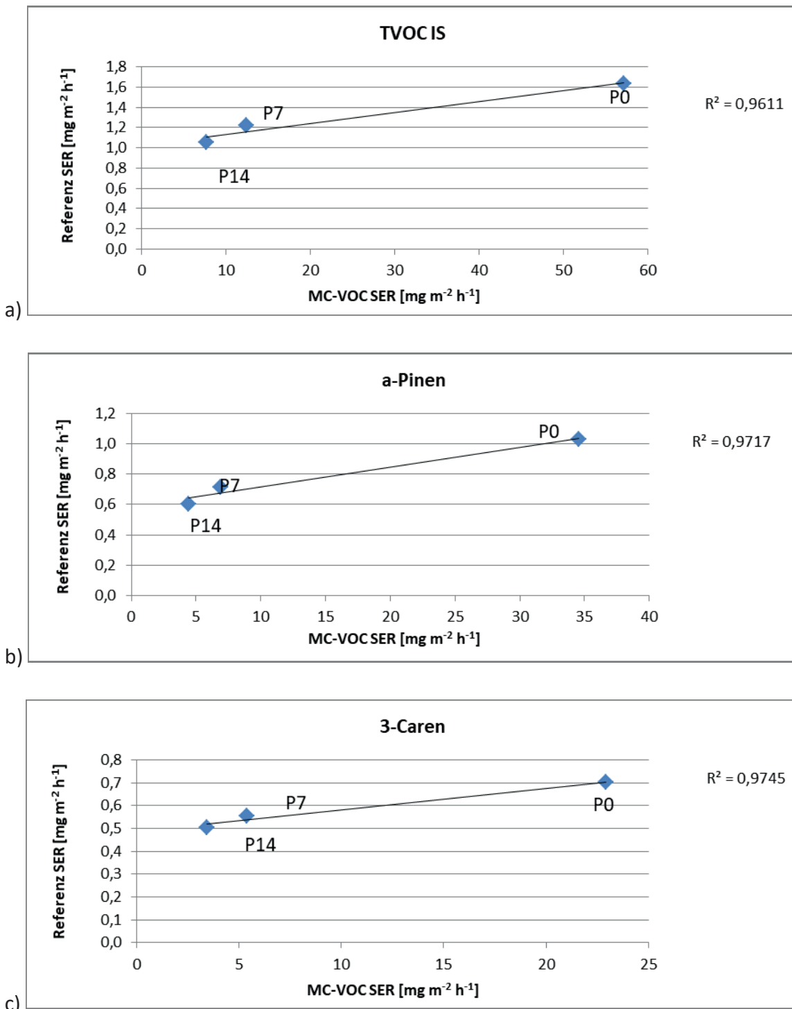
Abbildung 24: Korrelationen für TVOC IS (a), α-Pinen (b) und 3-Caren (c) zwischen MC-VOC und Referenztest aus Ergebnissen von nicht klimatisiertem und klimatisiertem Kiefern-Vollholz bei variierender Konditionierungsdauer in der Micro-Chamber
