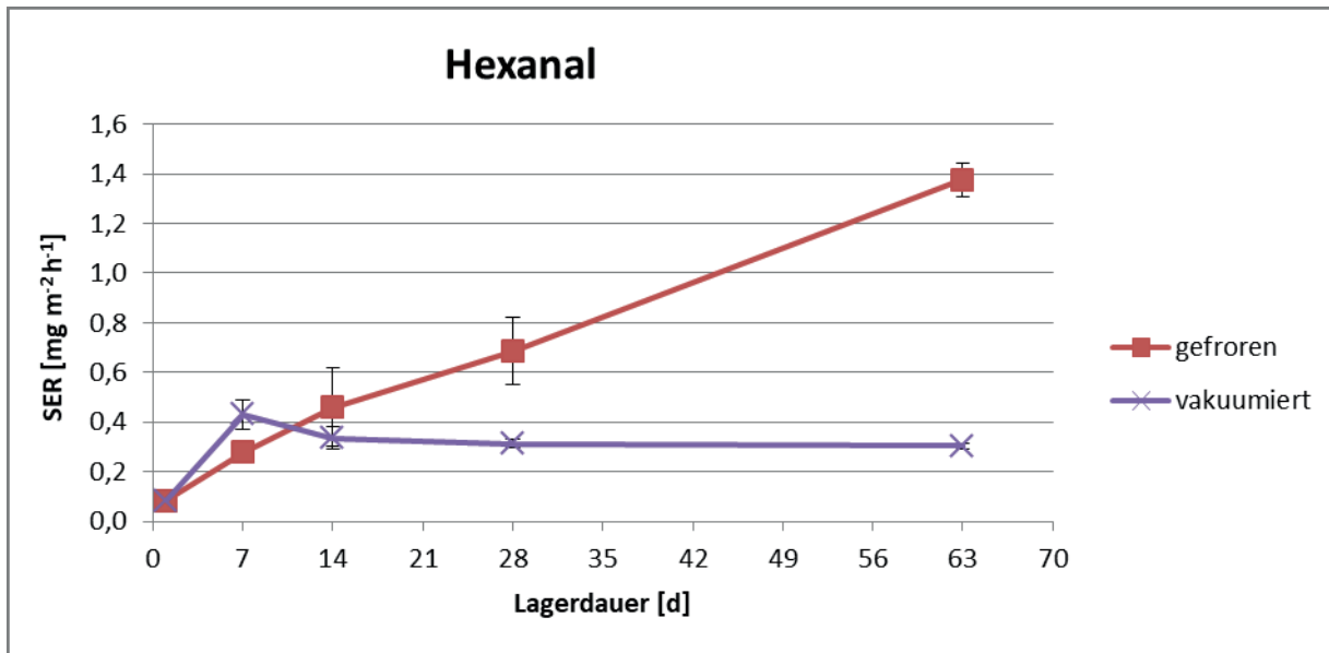
Abbildung A1: Hexanalemissionen aus gefrier gelagerter und vakuum gelagerter Kiefern-OSB im zeitlichen Verlauf der Lagerdauer, gemessen mit der MC-VOC
