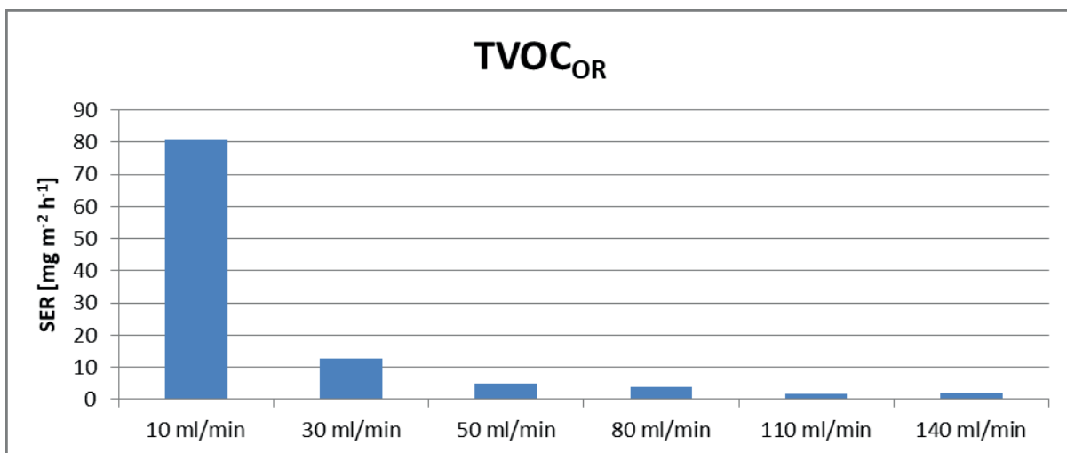
Abbildung A3: SER- \text{TVOC}_{\text{OR}} aus Kiefern-OSB bei variierendem Luftfluss während Konditionierung in der Micro-Chamber
