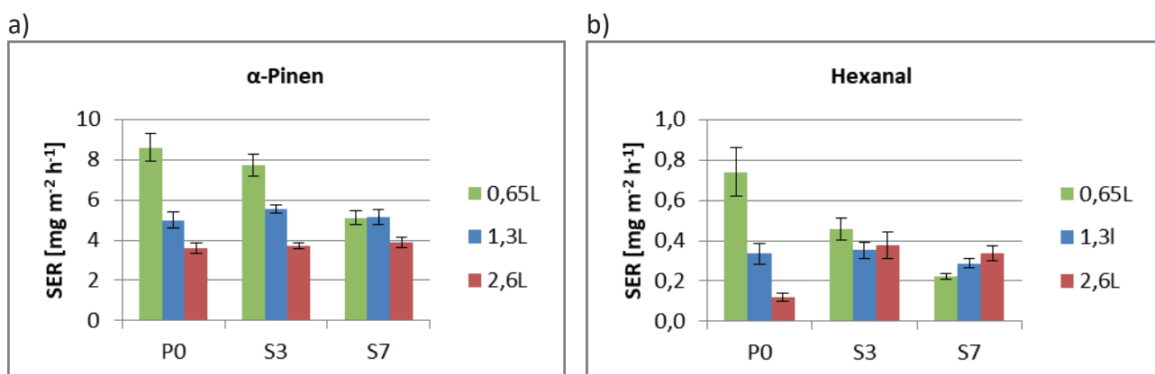
Abbildung 15: Emissionsraten aus ungestapelter und stapelgelagerter OSB der Dicke 22 mm, gemessen mit der MC-VOC
