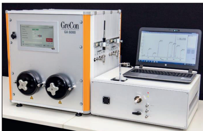
Abbildung 26: Prototyp GA-SPME-GC-FAIMS
