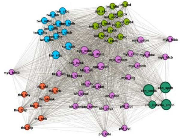
(d) Modularity groups
