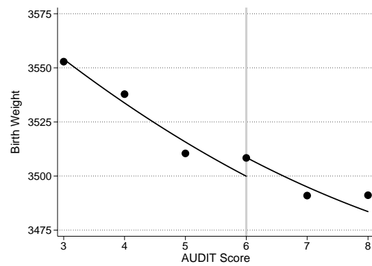
(d) 2nd order joint polynomial, AUDIT 3-8
