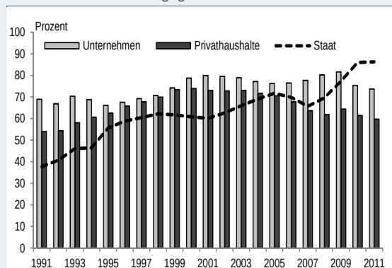
Abbildung 2: Sektorale Verschuldungsgrade 1991–2011
