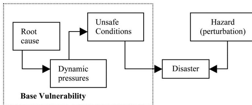
Figure 3: PAR model
