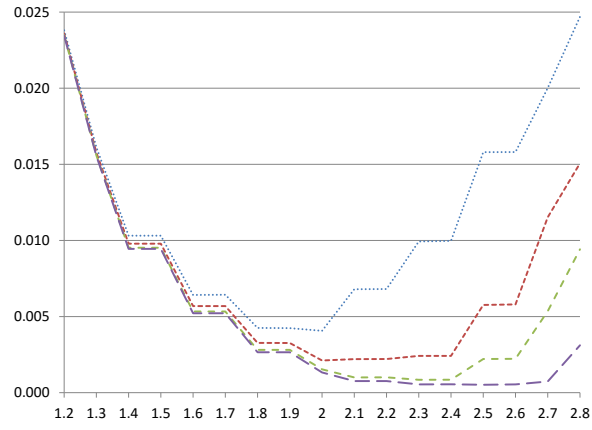
(a) V_0 \sim N(0, 0.1)
