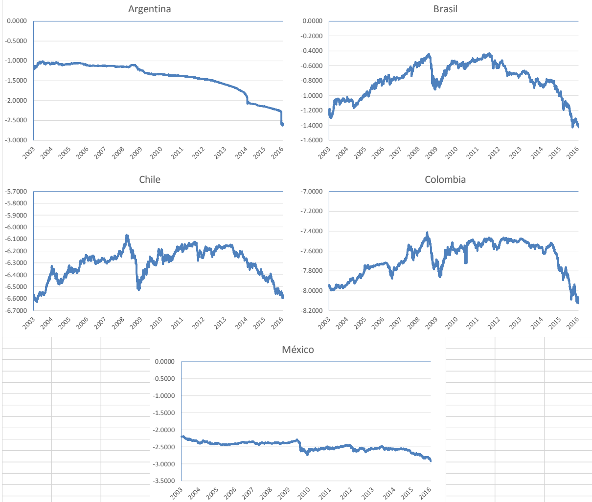
GRÁFICO A.2. TIPOS DE CAMBIO LATINOAMERICANOS, 05-08-2002 AL 22-01-2016
