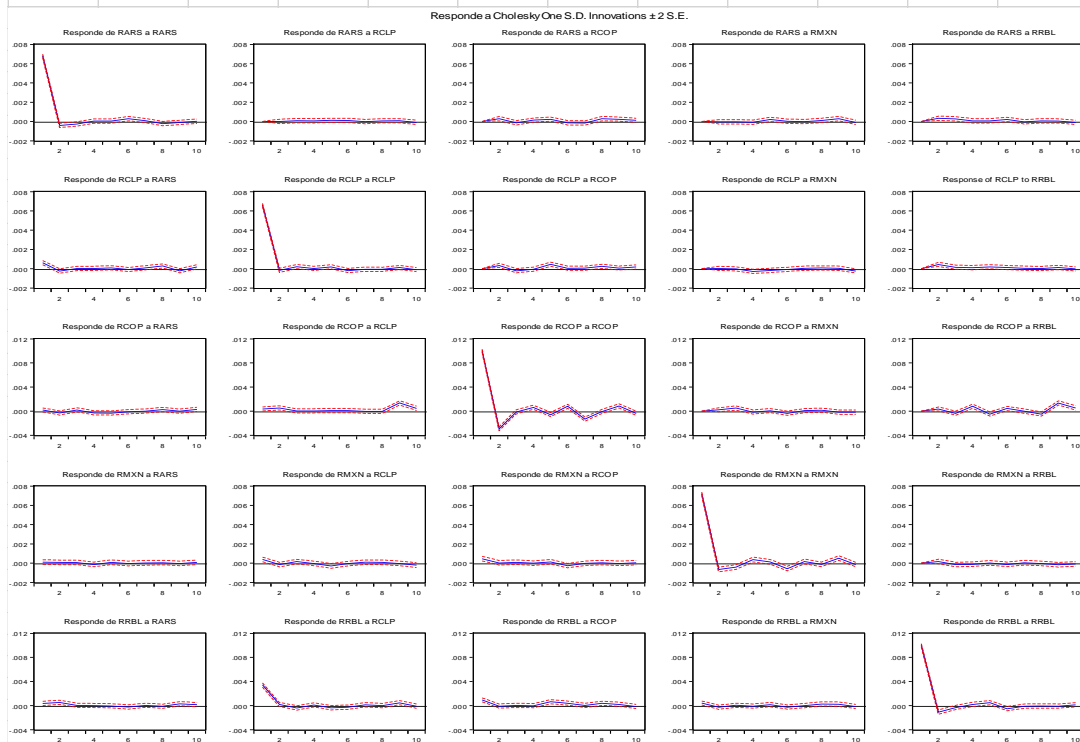
GRÁFICO 2. FUNCIONES DE IMPULSO-RESPUESTA PARA LAS SERIES LATINOAMERICANAS DE RENDIMIENTOS.
