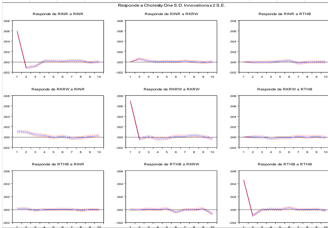
GRÁFICO 1. FUNCIONES DE IMPULSO-RESPUESTA PARA LAS SERIES ASIÁTICAS DE RENDIMIENTOS.
