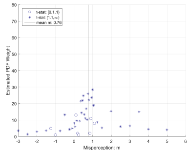
(d) Model III Dense Grid; f(m)
