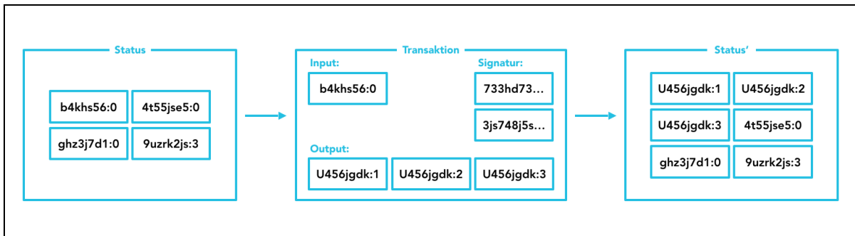
Abbildung 5: Bitcoin als Statusübergangssystem 43
