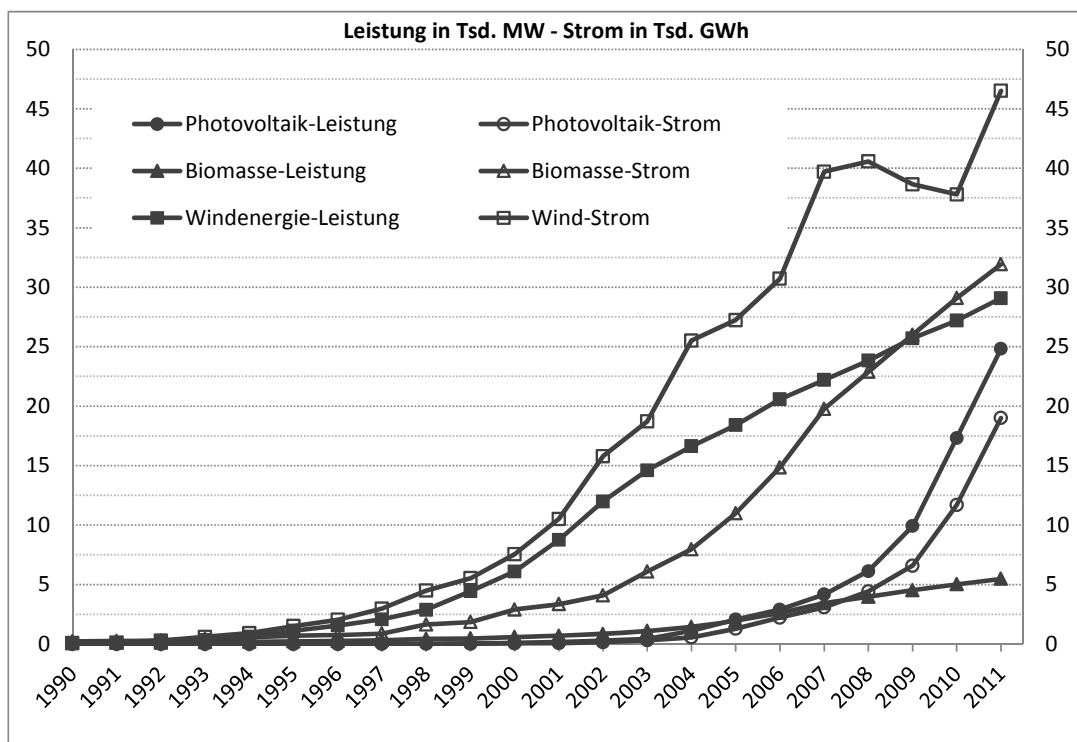
Abb. 6: Entwicklung der installierten Leistung und des Beitrags der erneuerbaren Energien zur Stromerzeugung 1990 bis 2011
