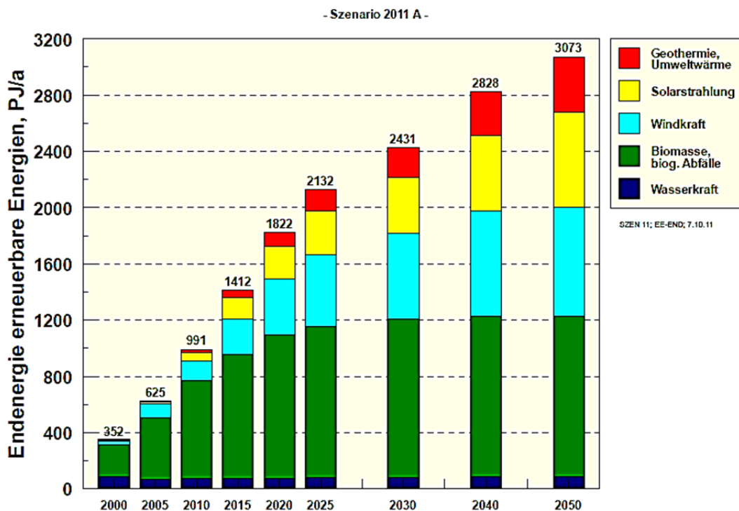
Abb. 11: Endenergiebeitrag der EE nach Energiequellen bis 2050
