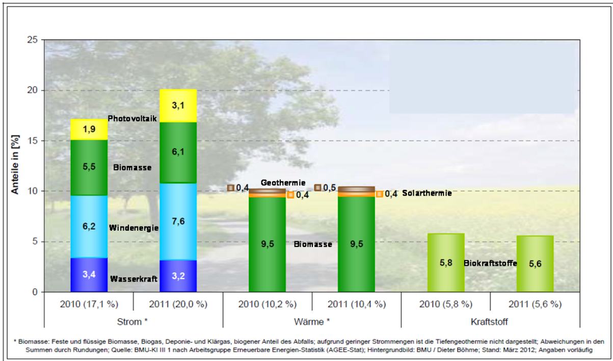
Abb. 5: Anteile der erneuerbare Energien-Sparten am Endenergieverbrauch 2010 und 2011
