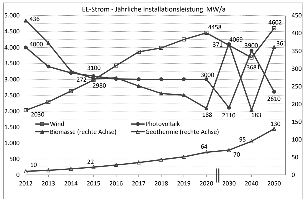
Abb. 12: Entwicklung der jährlichen Installationsleistung im Strombereich nach Sparten
