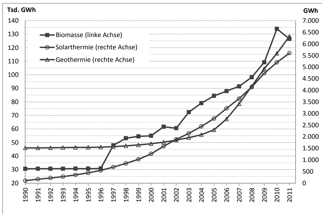
Abb. 7: Wärmebereitstellung durch erneuerbare Energien 1990 bis 2011
