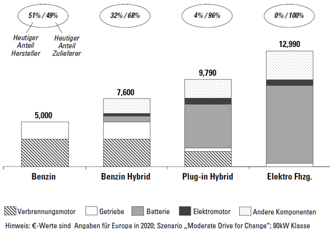
Abb. 17: Entwicklung von Wertschöpfungsstruktur und -umfang beim Antriebsstrang
