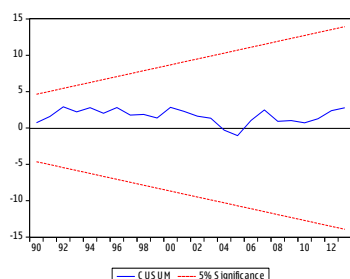
Fig. 1- CUSUM Test.
