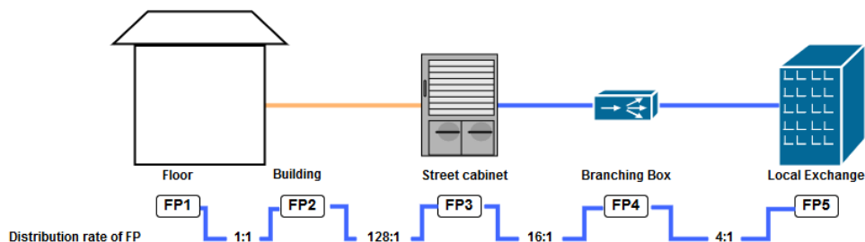
Fig 3. NGA network dimensioning model.
