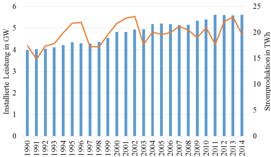
Abbildung 22: Installierte Leistung und Stromproduktion von Wasserkraft in Deutschland
