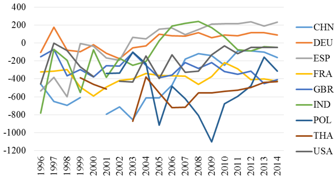
Abbildung 29: Spezialisierung ausgewählter Länder (RXA-Werte) bei Windkraftgeneratoren
