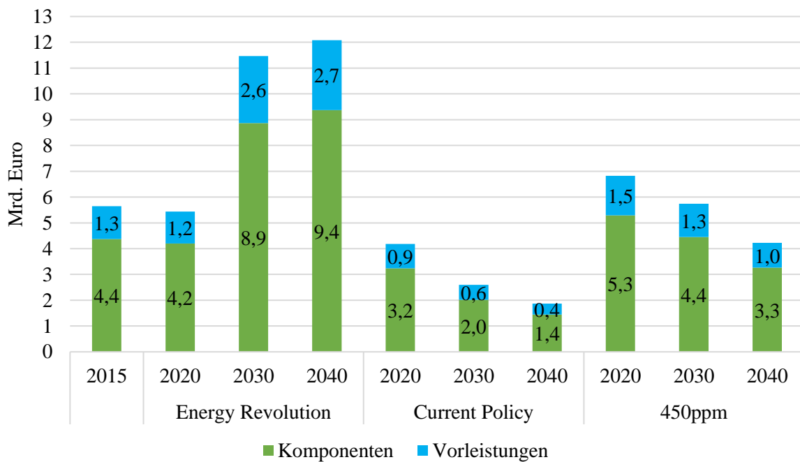
Abbildung 57: Aufteilung der Exporte in der Wind-Branche auf Komponenten und Vorleistungen in Mrd. Euro
