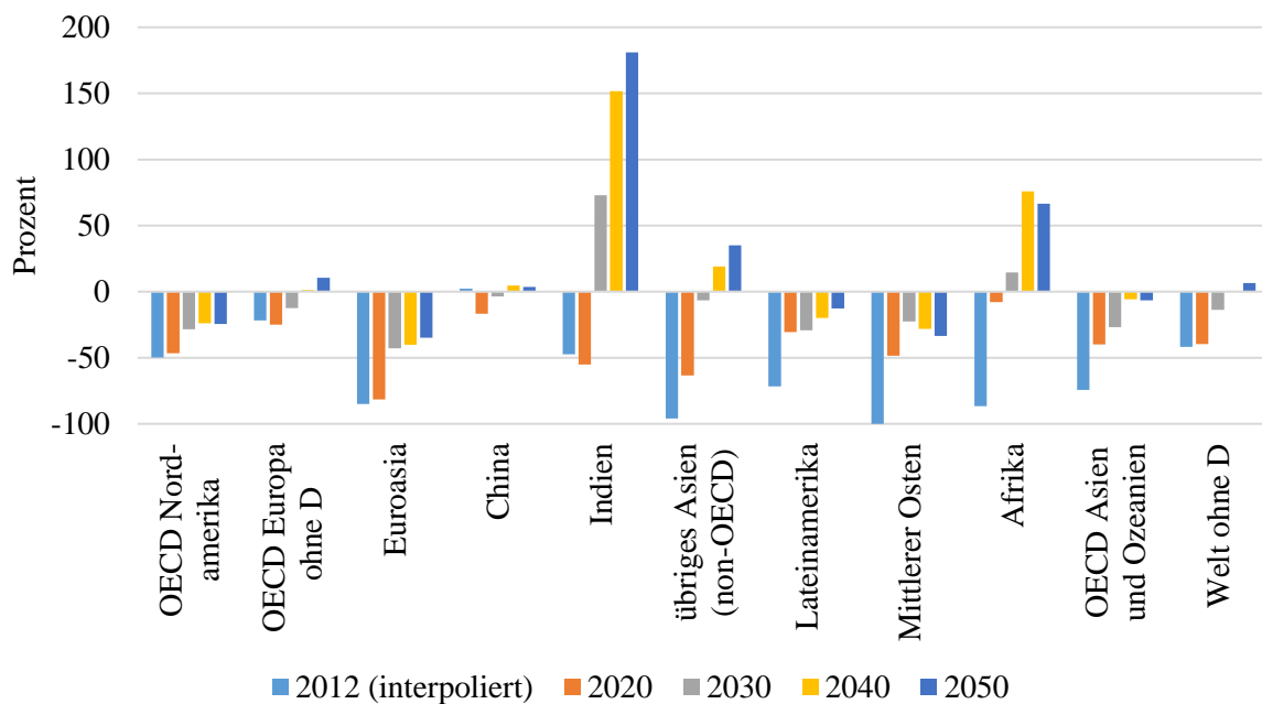
Abbildung 48: Prozentuale Abweichung der Ausbaupfade von Windkraft zwischen dem Energy-Revolution-Szenario von 2012 und 2015
