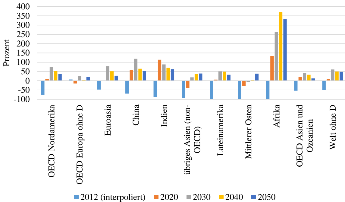
Abbildung 49: Prozentuale Abweichung der Ausbaupfade von Photovoltaik zwischen dem Energy-Revolution-Szenario von 2012 und 2015
