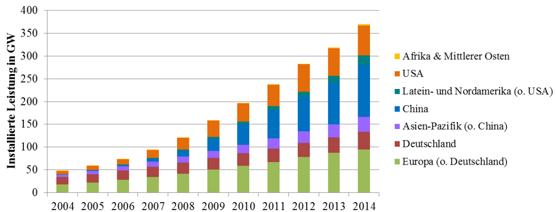
Abbildung 10: Weltweit kumulierte installierte Wind-Leistung in GW
