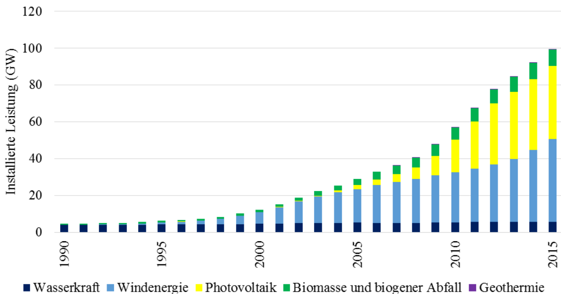
Abbildung 8: Installierte Leistung zur Strombereitstellung aus erneuerbaren Energien in Deutschland in den Jahren 1990 bis 2014
