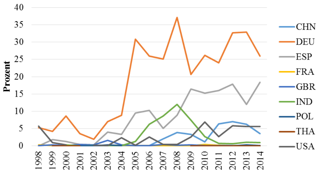
Abbildung 26: Welthandelsanteile ausgewählter Länder bei Windkraftgeneratoren
