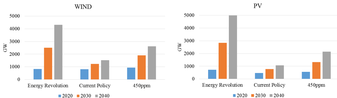
Abbildung 50: Zusammenschau der Ausbauszenarien für Wind Onshore und Photovoltaik
