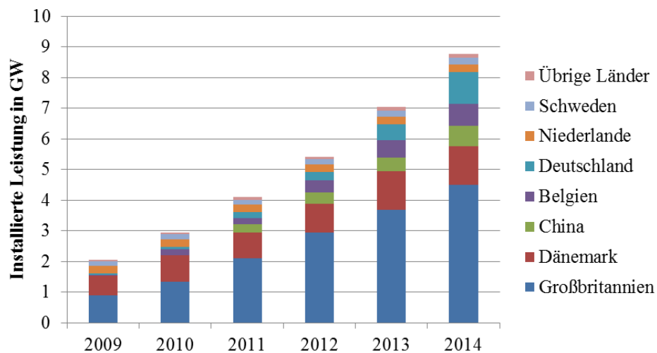
Abbildung 11: Weltweit installierte Offshore-Wind-Leistung in GW
