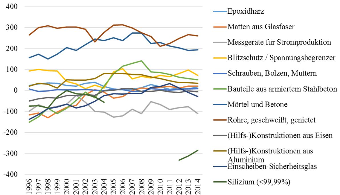
Abbildung 46: Außenhandelsspezialisierung (RCA-Werte) für Deutschland bei Vorleistungen für Wind, Photovoltaik und Wasserkraft
