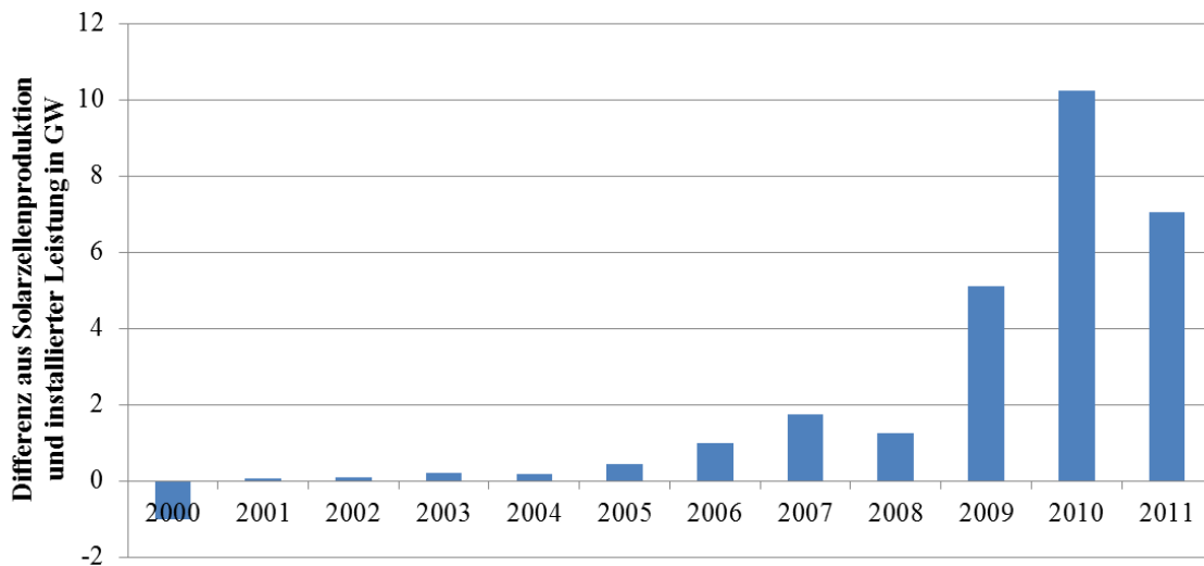
Abbildung 20: Differenz aus jährlicher weltweiter Solarzellenproduktion und installierter Photovoltaik-Leistung in den Jahren 2000 bis 2011 in GW
