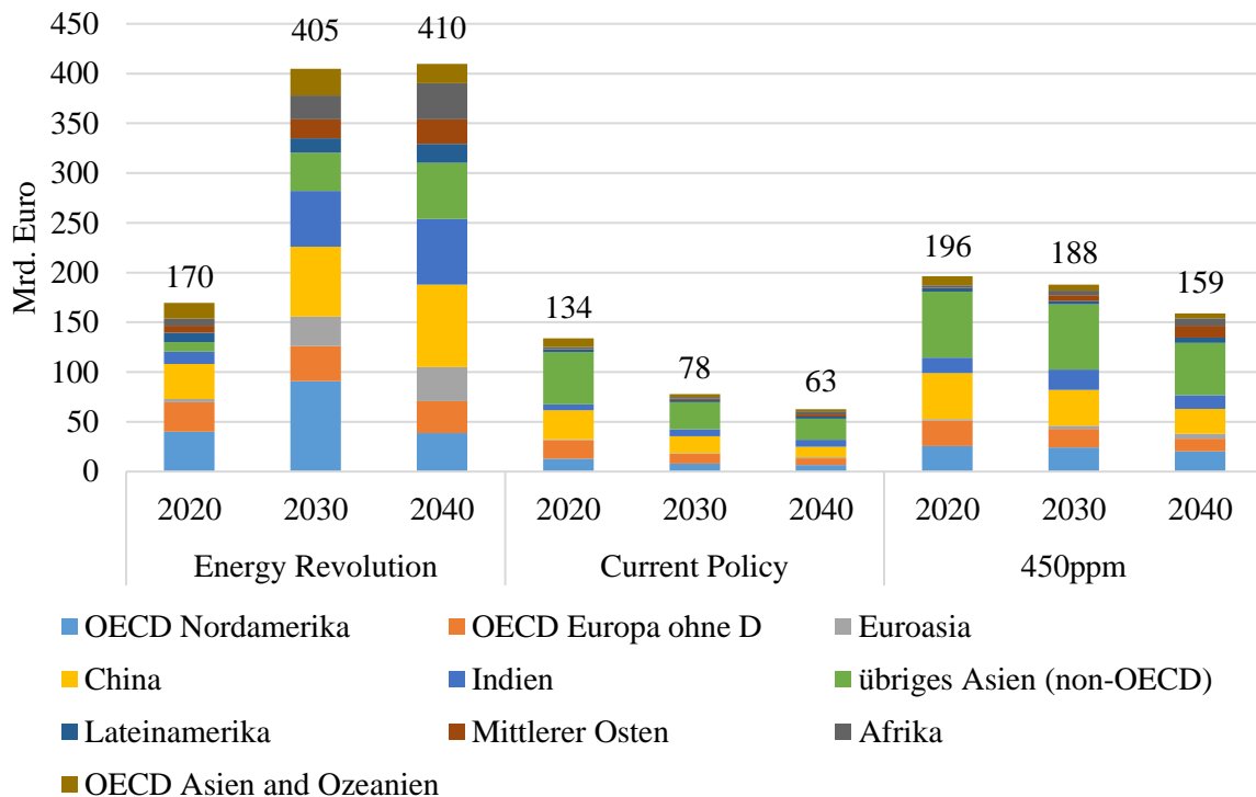
Abbildung 52: Jährliche Investitionen für die Technologien Wind Onshore und Photovoltaik im Energy-Revolution-Szenario, Current-Policy-Szenario und 450ppm Szenario
