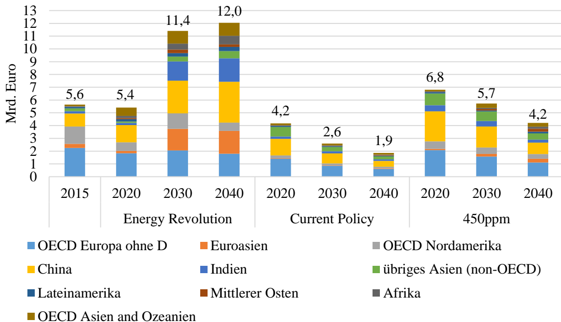
Abbildung 58: Exporte deutscher Unternehmen in der Wind-Branche nach Regionen in Mrd. Euro
