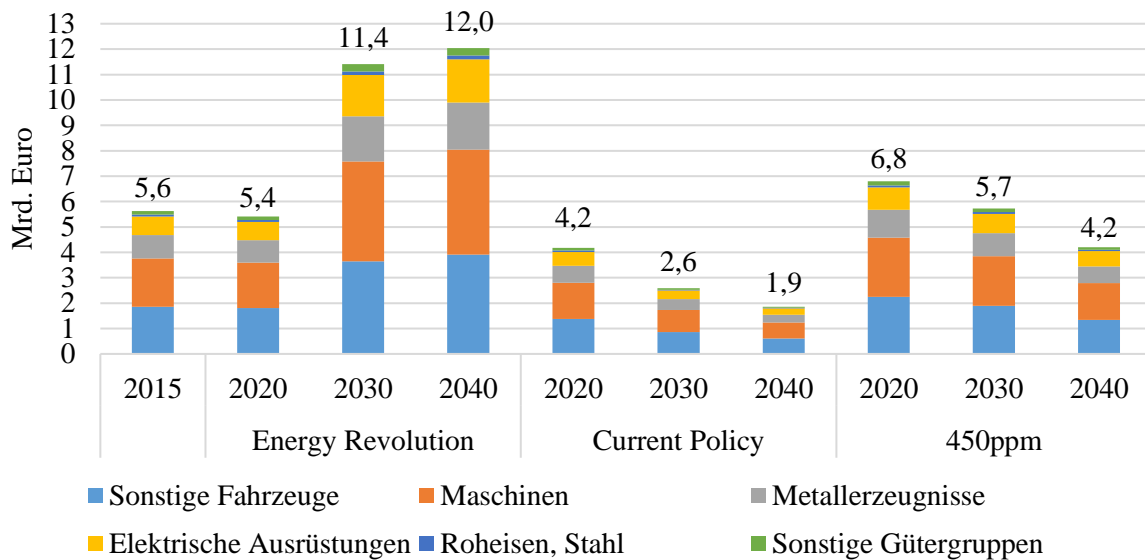
Abbildung 56: Exporte deutscher Unternehmen in der Wind-Branche nach Gütergruppen in Mrd. Euro
