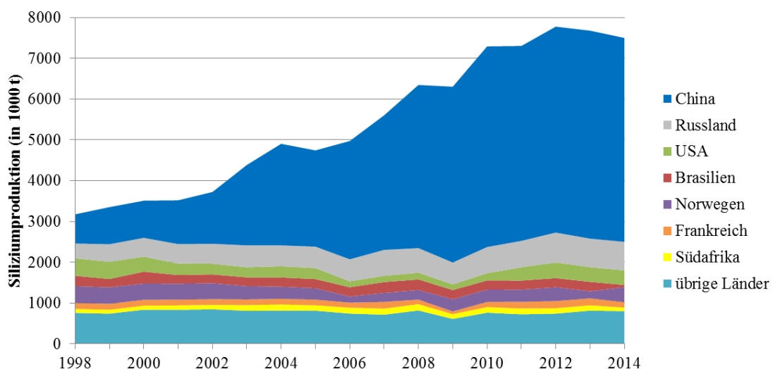
Abbildung 12: Siliziumproduktion in den bedeutendsten Produktionsländern von 1998 bis 2014 (in 1000 t)
