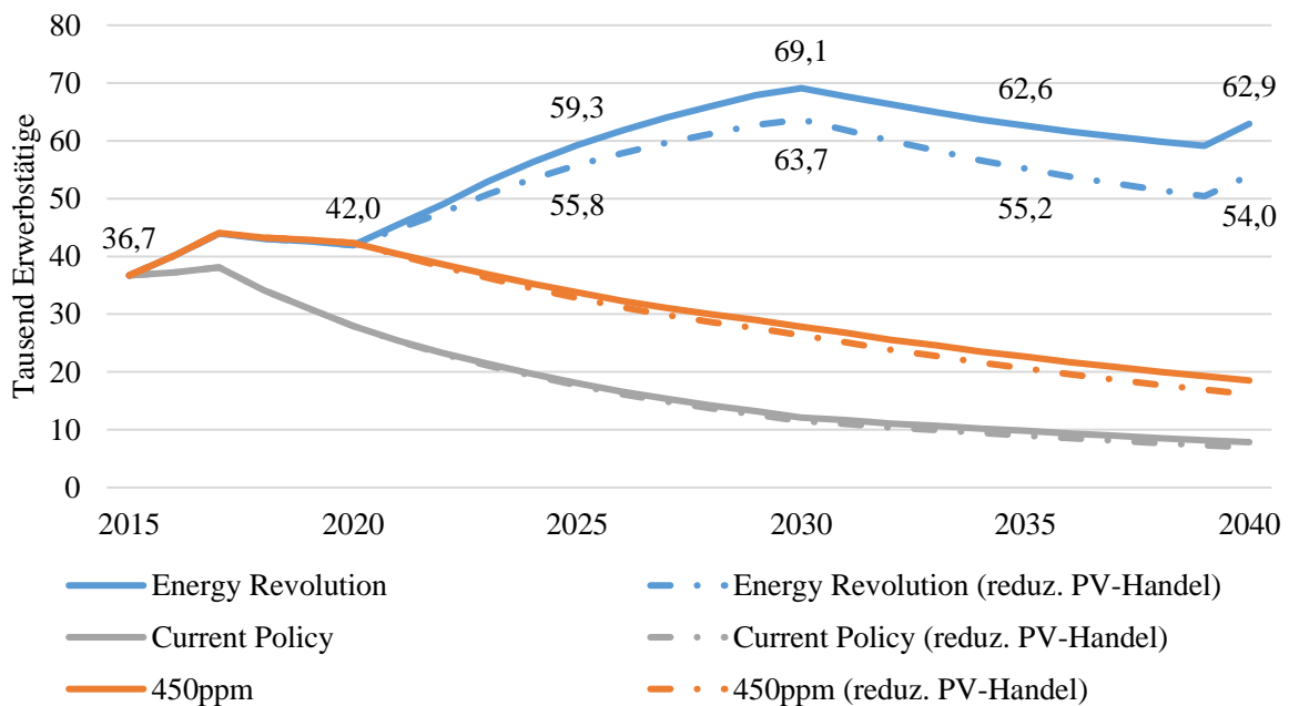
Abbildung 69: Auswirkungen eines reduzierten PV-Handels auf die Beschäftigung
