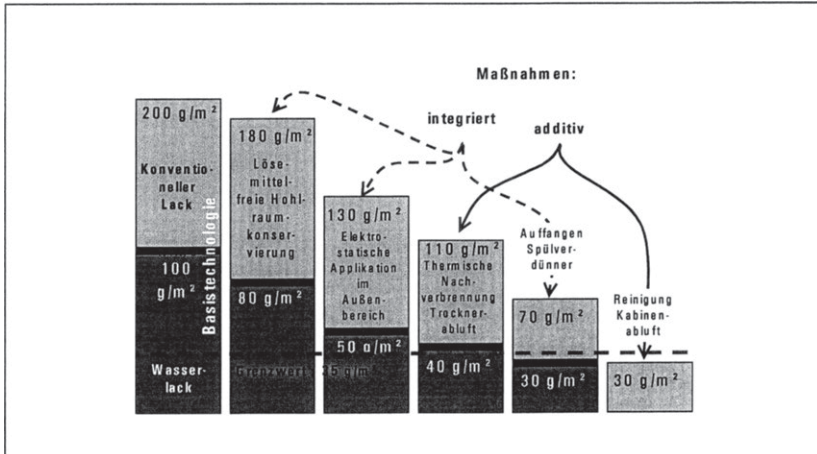
Abbildung 7: VOC-Reduktion
