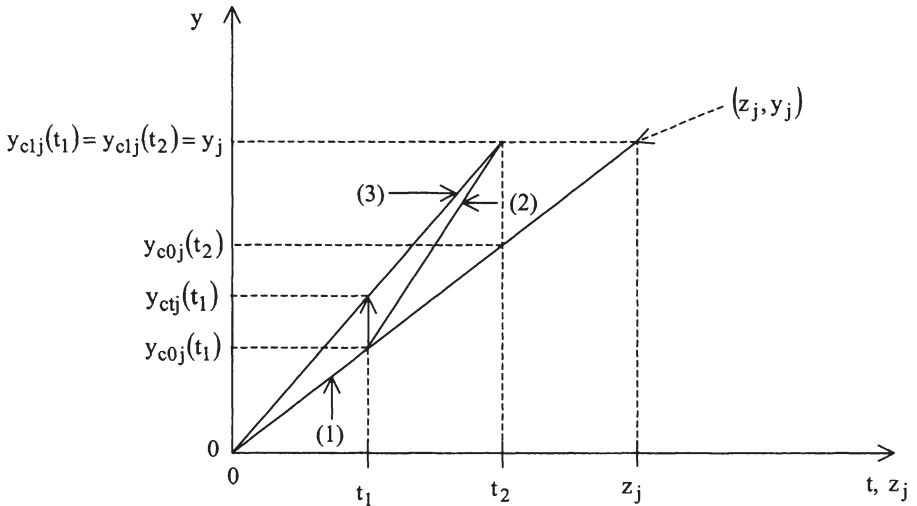
Abbildung 3.15: Verletzung der ersten Konkavitätsbedingung in (3.108)
