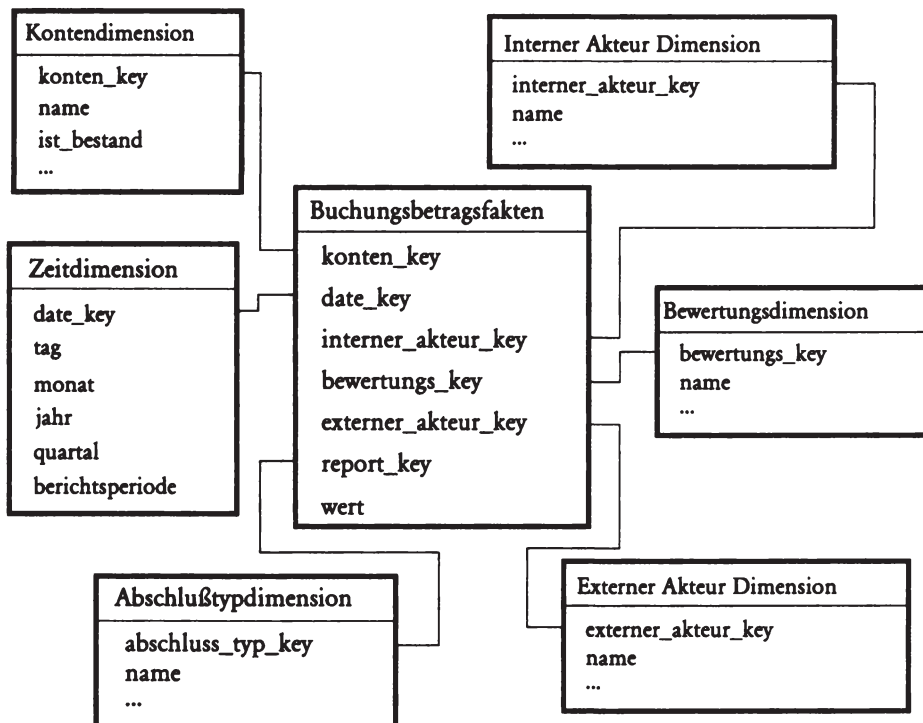
Abb. 10: PAIS-Datenmodell 1. Stufe
