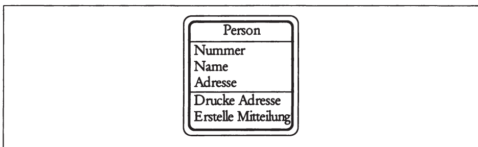
Abbildung 5-2: Schematische Darstellung der Klasse Person.
