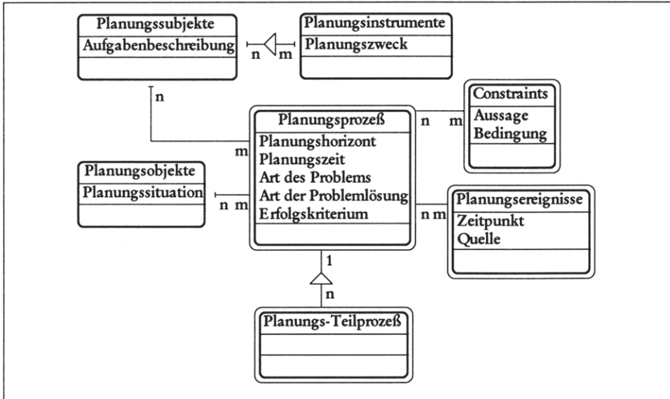
Abbildung 6-12: Allgemeines Objektmodell des Planungsprozesses.
