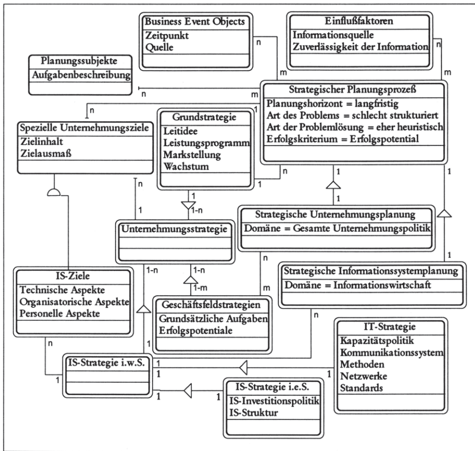
Abbildung 6-13: Objektmodell des integrierten strategischen Planungsprozesses.
