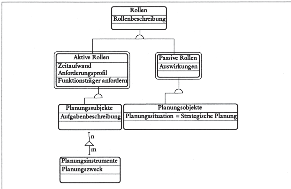
Abbildung 6-6: Rollen der integrierten strategischen Planung.
