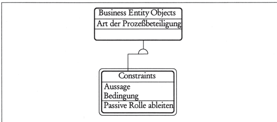
Abbildung 5-22: Die Klasse Constraints.
