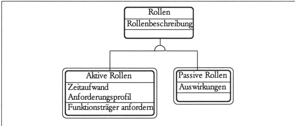
Abbildung 5-19: Die Klasse Rollen mit ihren Unterklassen.
