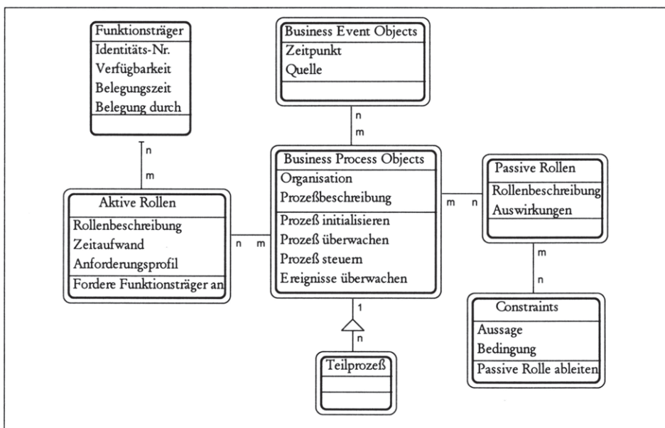
Abbildung 5-27: Business Process Objects und ihre Objektbeziehungen. 364
