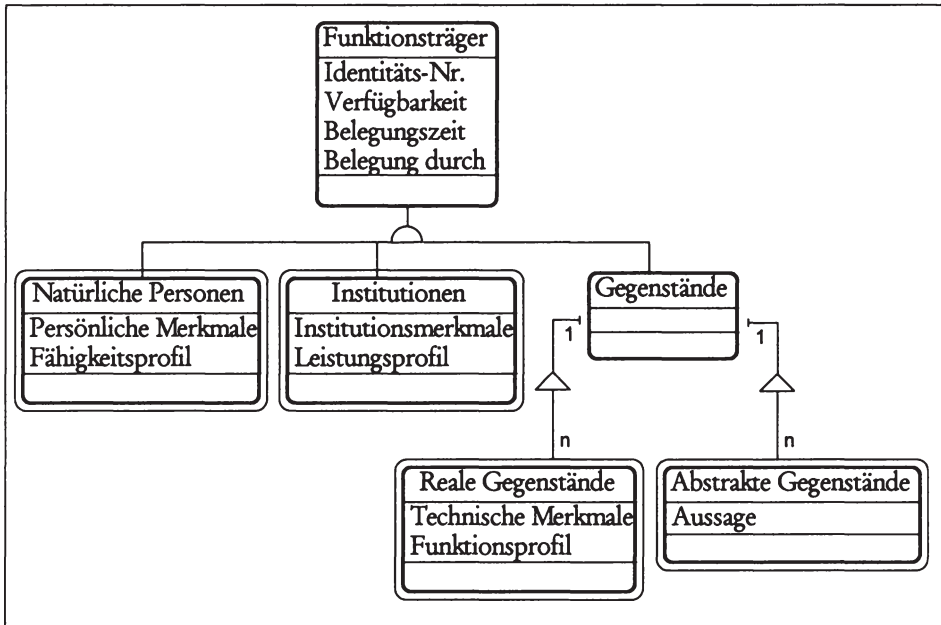
Abbildung 5-18: Die Klasse Funktionsträger mit ihren Unterklassen.
