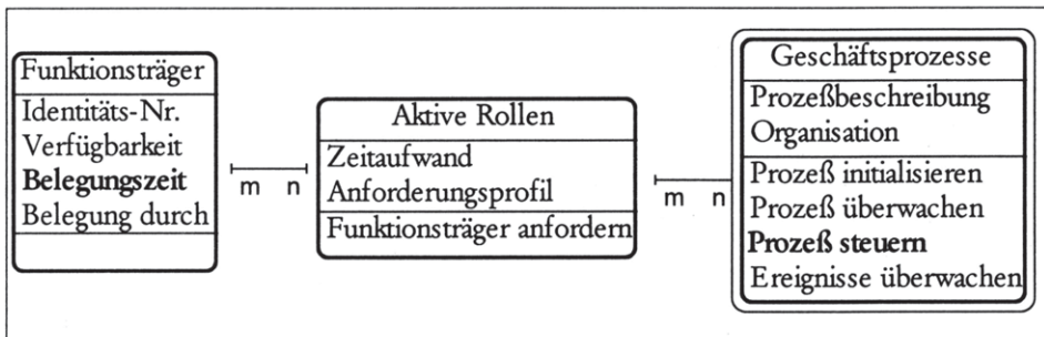
Abbildung 5-20: Der Zusammenhang von Funktionsträger, aktiver Rolle und Prozeß.
