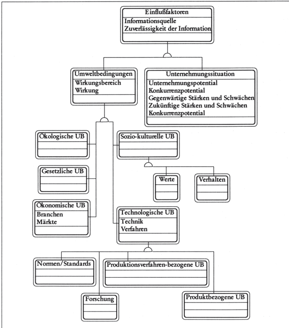
Abbildung 6-10: Objektorientierte Darstellung der Einflussfaktoren der strategischen Planung.
