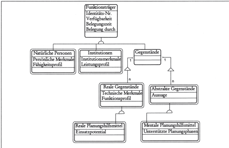
Abbildung 6-5: Funktionsträger der integrierten strategischen Planung.
