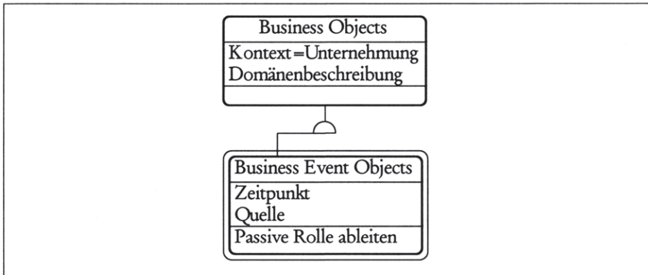
Abbildung 5-23: Die Klasse Business Event Objects.
