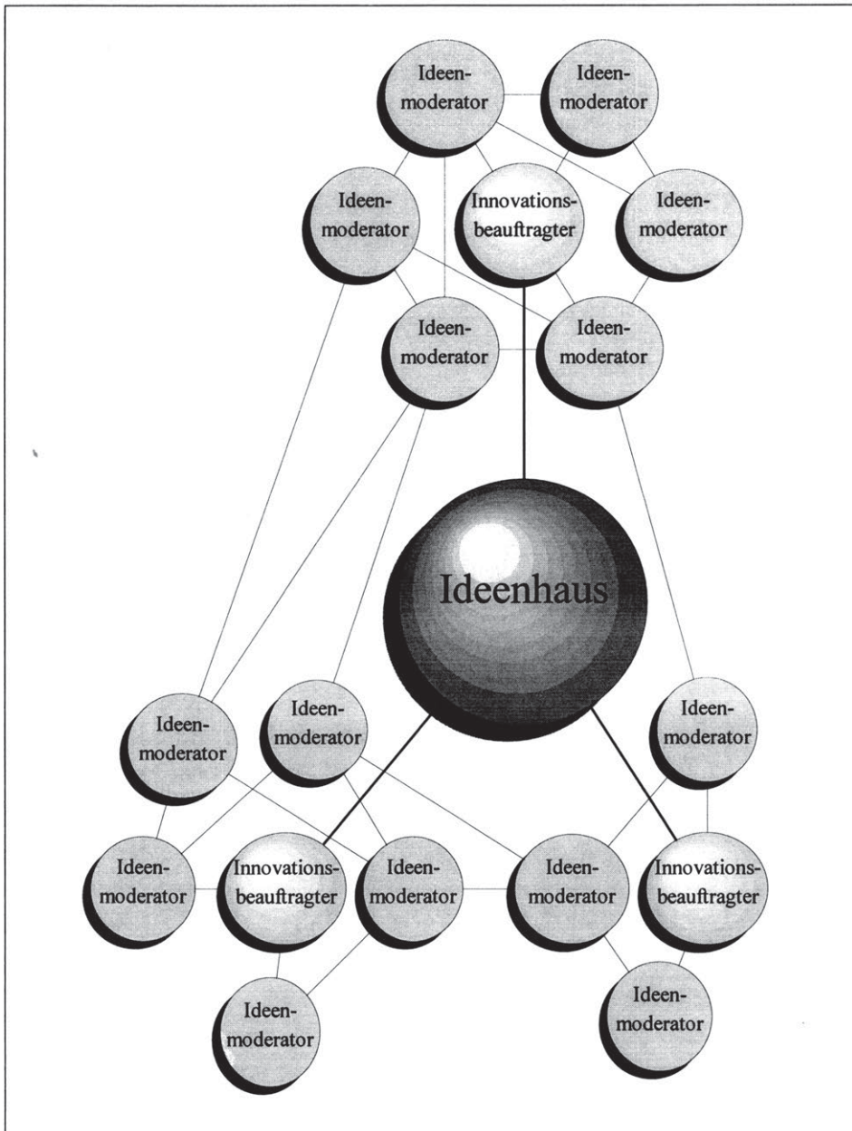
Abbildung 6-1: Ideenhaus. 376
