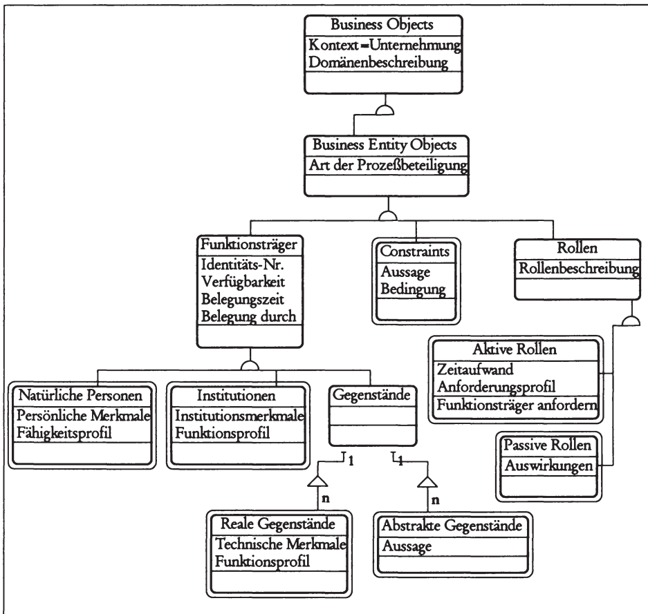
Abbildung 5-17: Arten von Business Entity Objects. 349
