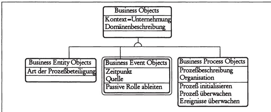
Abbildung 5-16: Spezielle Arten von Business Objects. 346
