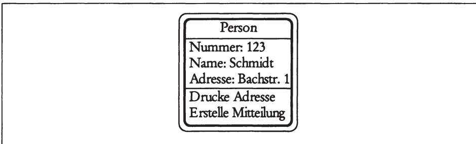
Abbildung 5-1: Schematische Darstellung des Objekts Person. 280
