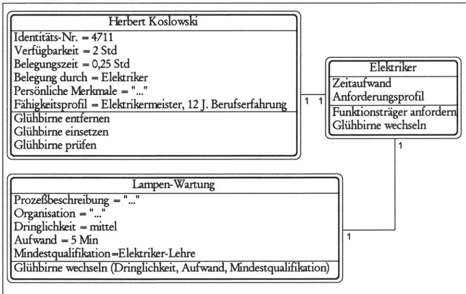
Abbildung 5-21: Beispiel „Lampen-Wartung“.
