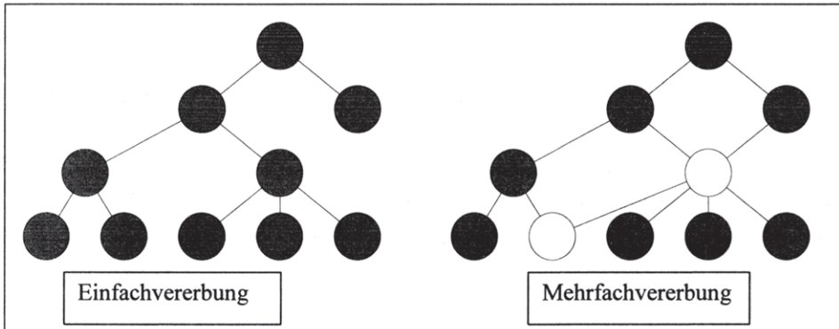
Abbildung 5-4: Vererbungsformen. 286
