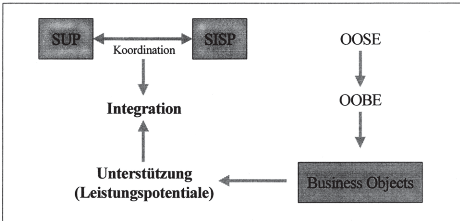
Abbildung 1-1: Lösungsansatz.
