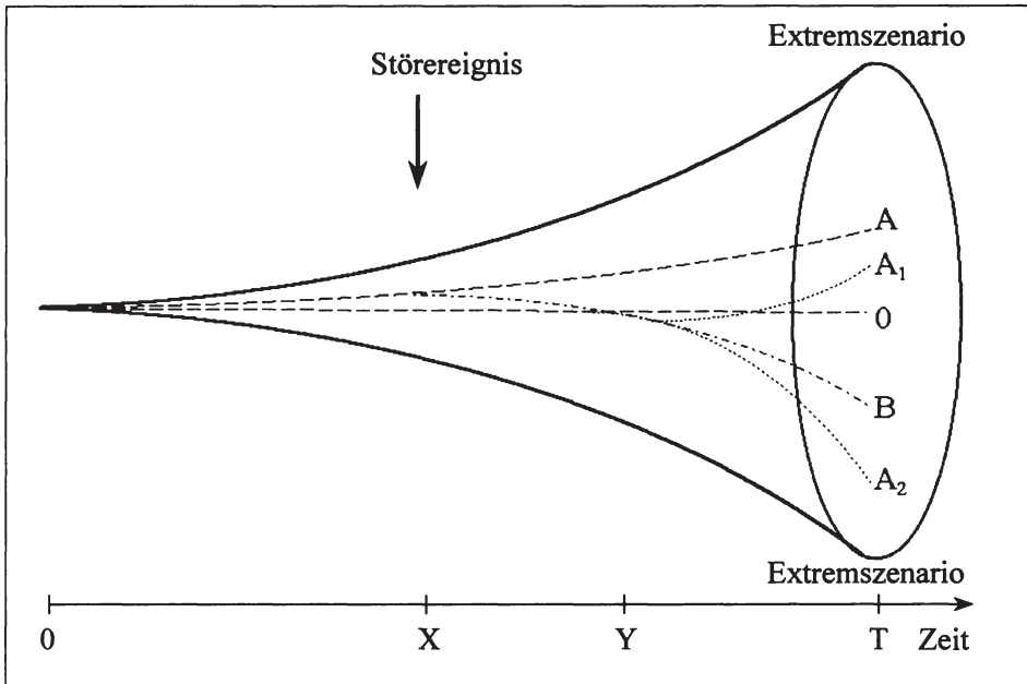
Abbildung 2-7: Szenario-Trichter. 100
