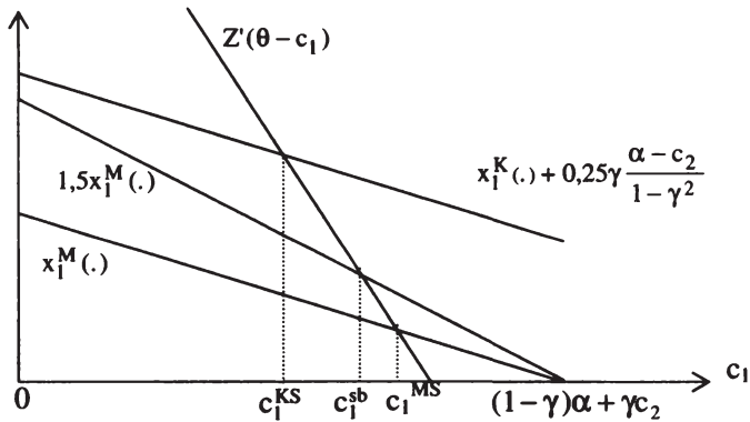
Abbildung 3.19: Überinvestition in kostenreduzierenden Maßnahmen bei Kollusion
