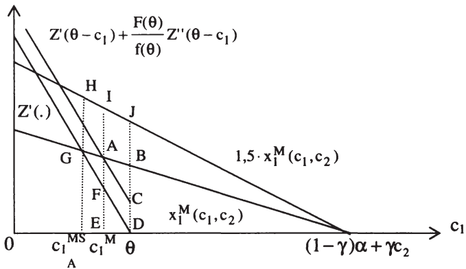
Abbildung 3.11: Kostenreduktion im Monopol bei unvollständiger Information
