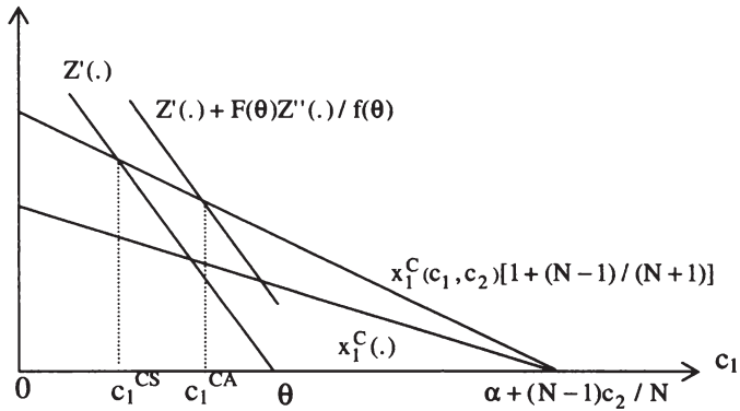
Abbildung 4.2: Grenzkosten bei Cournotwettbewerb und unvollständiger Information
