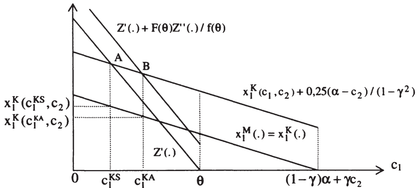
Abbildung 3.23: Reduktion der Grenzkosten bei Kollusion und unvollständiger Information
