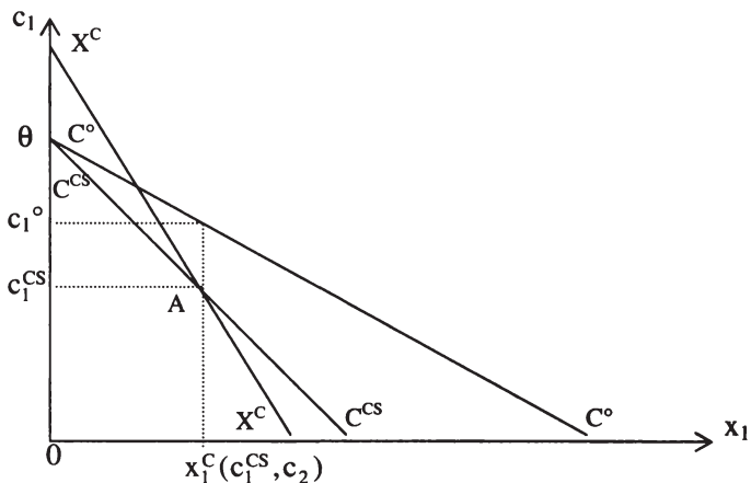
Abbildung 3.35: X-Ineffizienz bei Cournotwettbewerb und vollständiger Information
