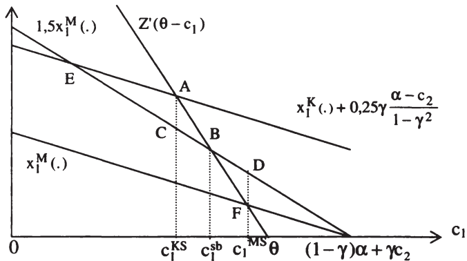
Abbildung 3.18: Überinvestition in kostenreduzierende Maßnahmen bei Kollusion
