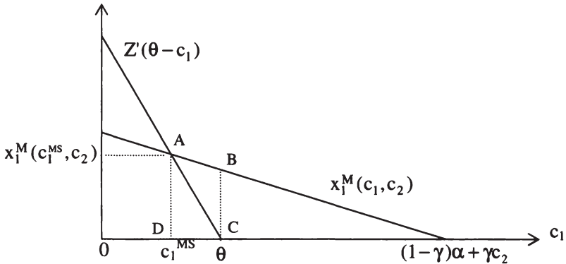
Abbildung 3.3: Reduktion der Grenzkosten im Monopol bei vollständiger Information
