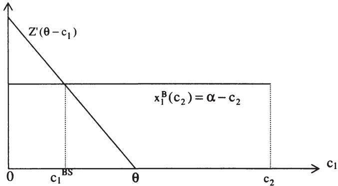
Abbildung 4.3: Grenzkosten bei Verdrängungswettbewerb und vollständiger Information
