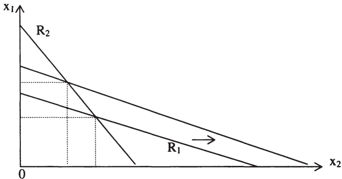
Abbildung 3.31: Reaktionskurven bei Cournotwettbewerb
