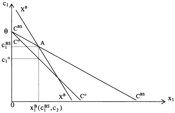
Abbildung 3.51: X-Ineffizienz bei Bertrandwettbewerb und vollständiger Information
