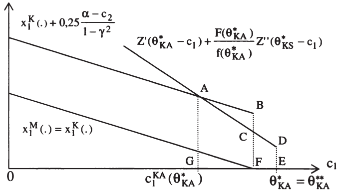
Abbildung 3.30: Keine Kostenreduktion bei Kollusion und unvollständiger Information
