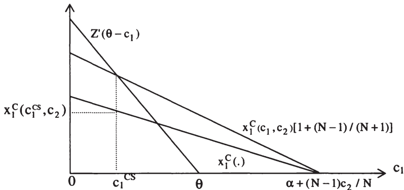
Abbildung 4.1: Grenzkosten bei Cournotwettbewerb und vollständiger Information
