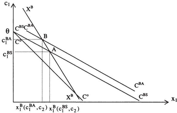
Abbildung 3.54: X-Ineffizienz bei Bertrandwettbewerb und unvollständiger Information
