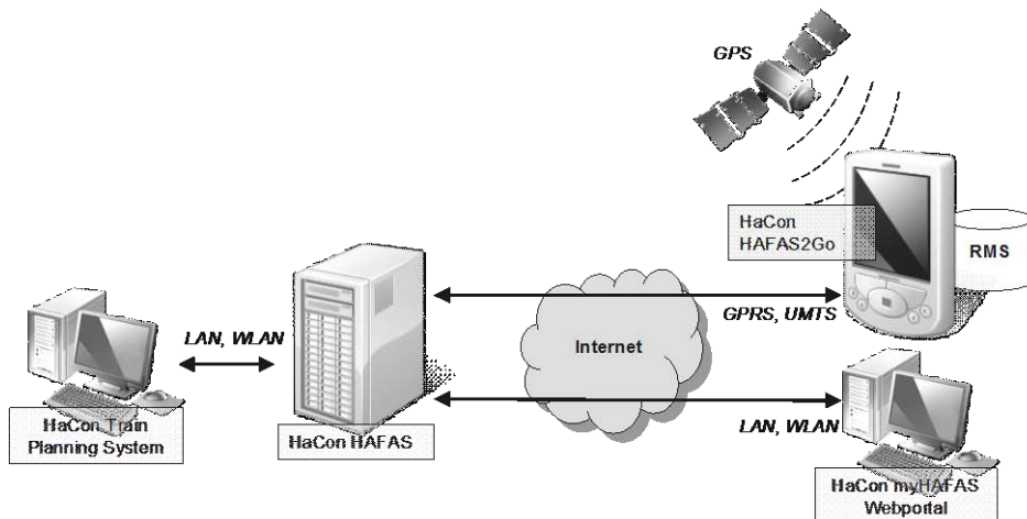
Abbildung 43: Architektur des Fahrplanauskunftssystems der HaCon
