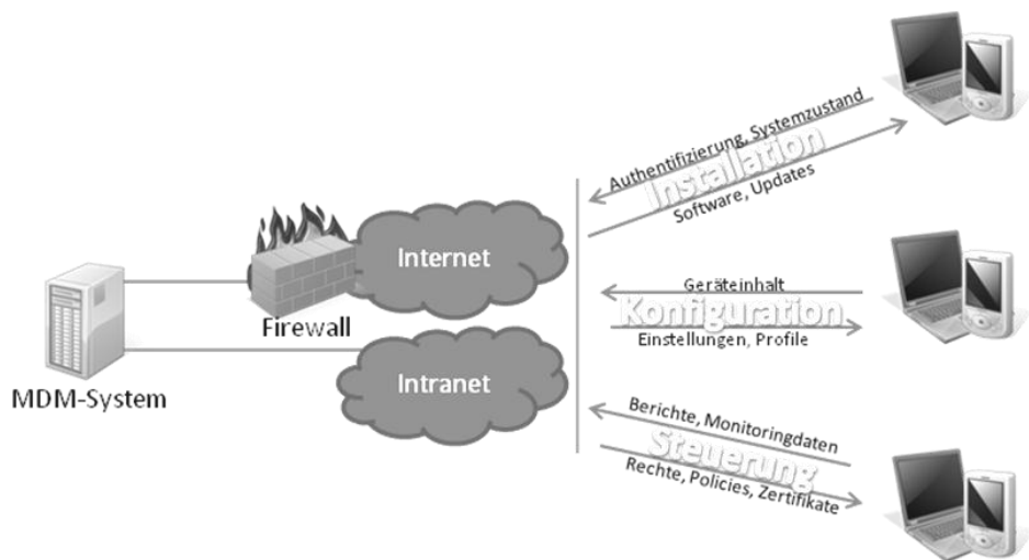
Abbildung 67: Schematischer Aufbau eines MDM-Systems 84
