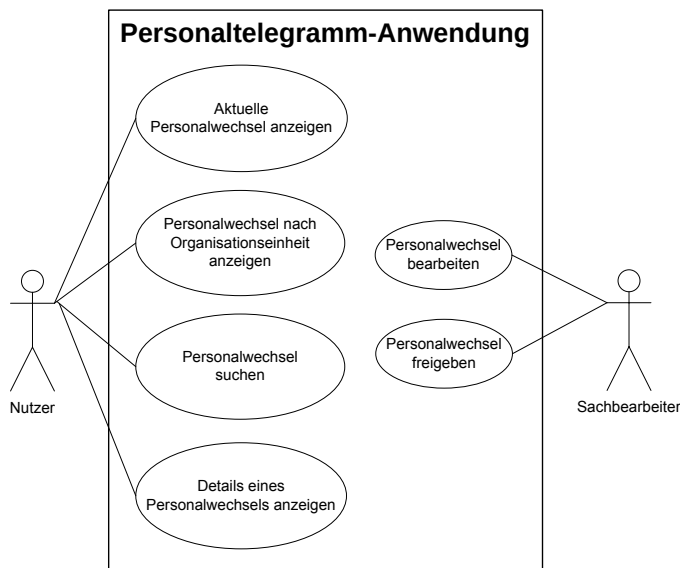
Abbildung 95: Anwendungsfalldiagramm der Personaltelegramm-Anwendung
