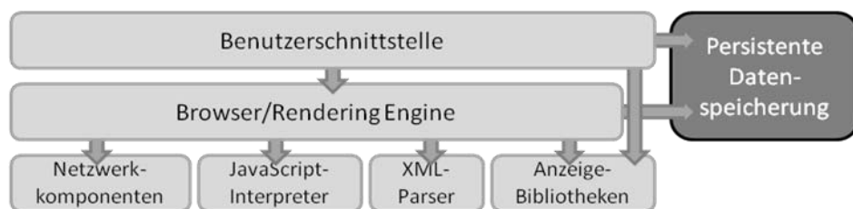
Abbildung 12: Webbrowser-Referenzarchitektur 20
