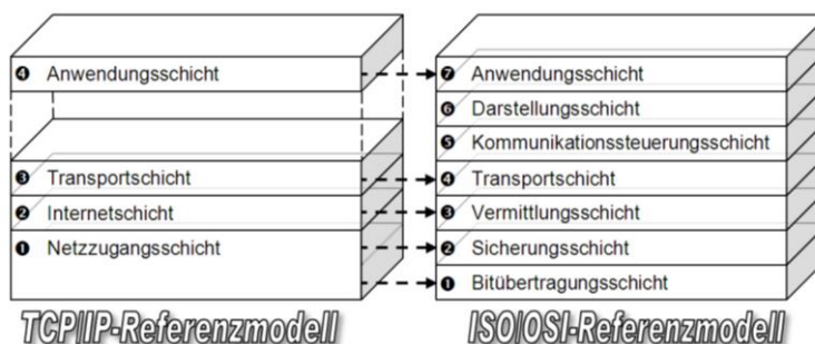
Abbildung 6: Gegenüberstellung von TCP/IP- und ISO/OSI-Referenzmodell
