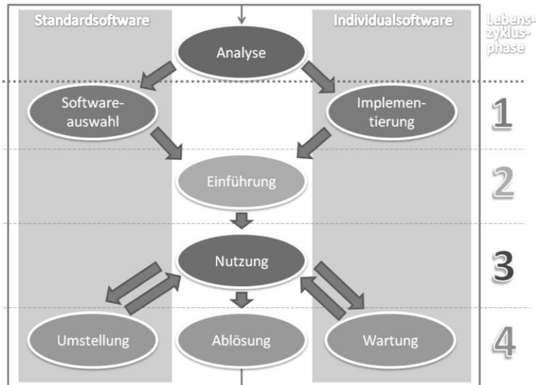
Abbildung 27: Vereinfachter Software-Lebenszyklus 41
