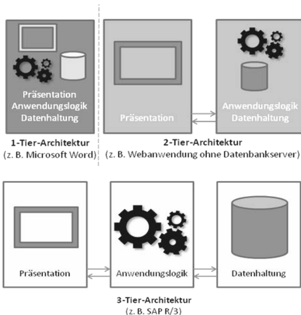
Abbildung 75: Beispielhafte n-Tier-Architekturen
