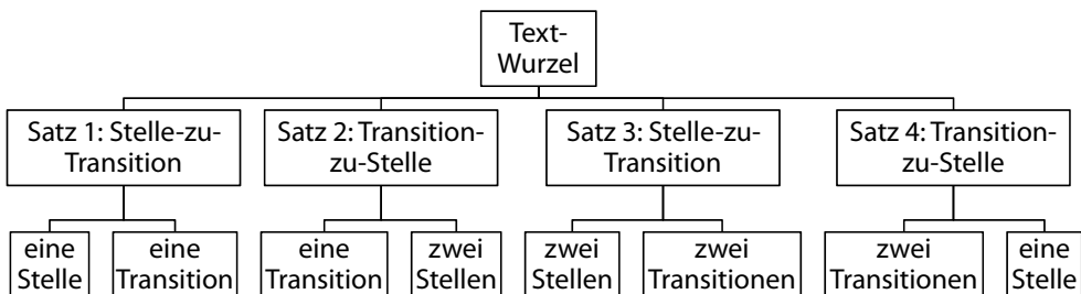
Abb. 4.3: Beispielsatz in eine Baumstruktur überführt
