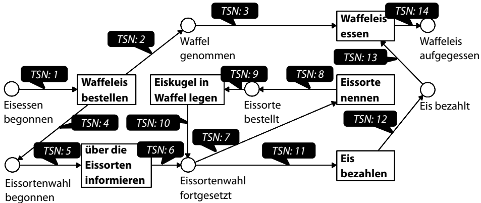
Abb. 4.12: Beispielnummerierung der Tiefsuchnummer zu Abb. 4.10
