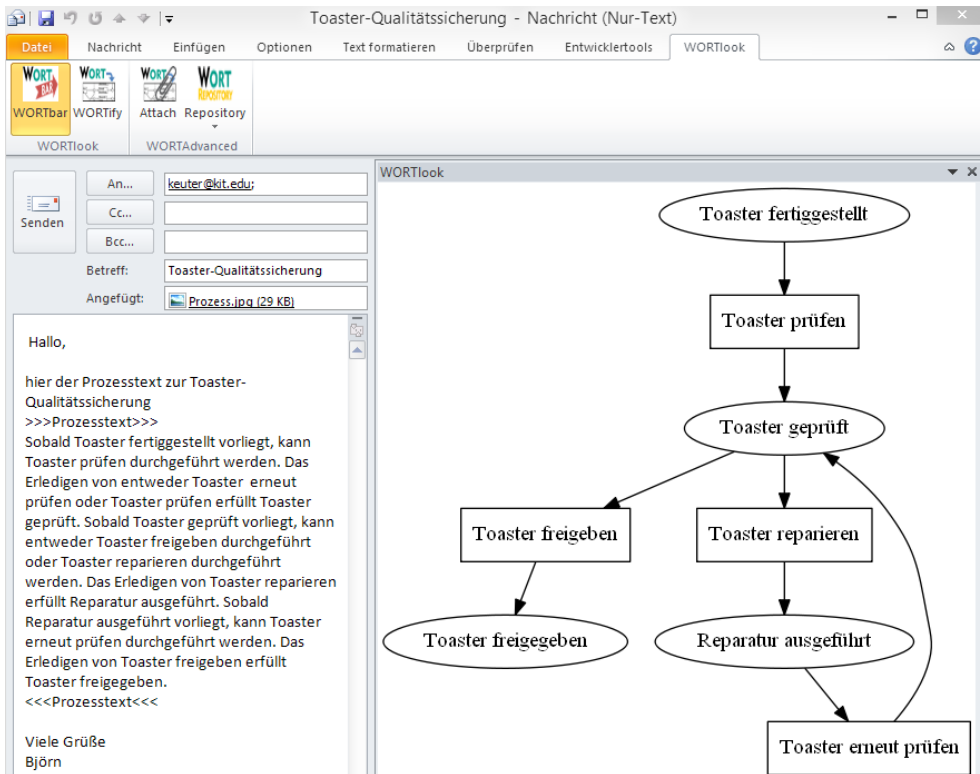
Abb. 6.10: E-Mail mit Prozesstext und umgebenden Nachrichtentext
