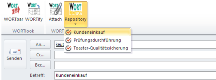
Abb. 6.9: Prozesstext-Repository
