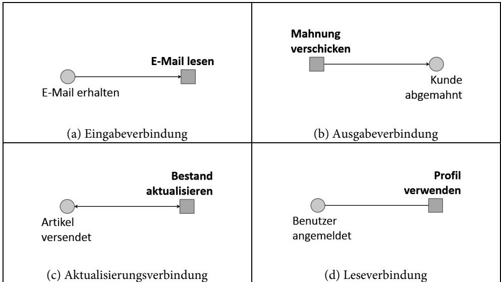
Abb. 5.2: Einfache Verbindungen
