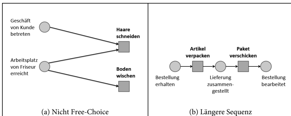
Abb. 5.5: Spezielle Ablaufstrukturen
