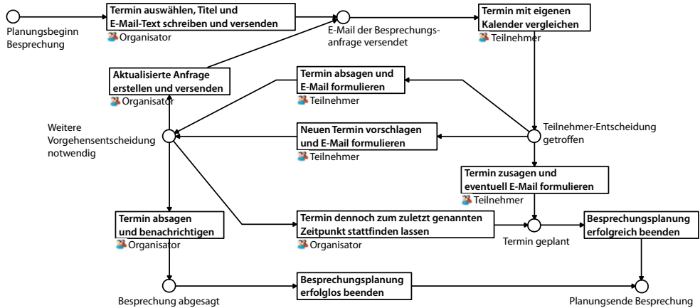
Abb. 2.11: Prozessmodell Besprechungsanfrage
