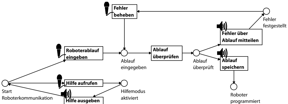
Abb. 3.7: Szenario 3 – Dialogbasierte Steuerung von Robotern
