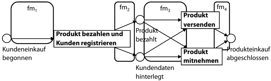
Abb. 4.6: Elemente der Satzkanzenmenge FM des Beispiels
