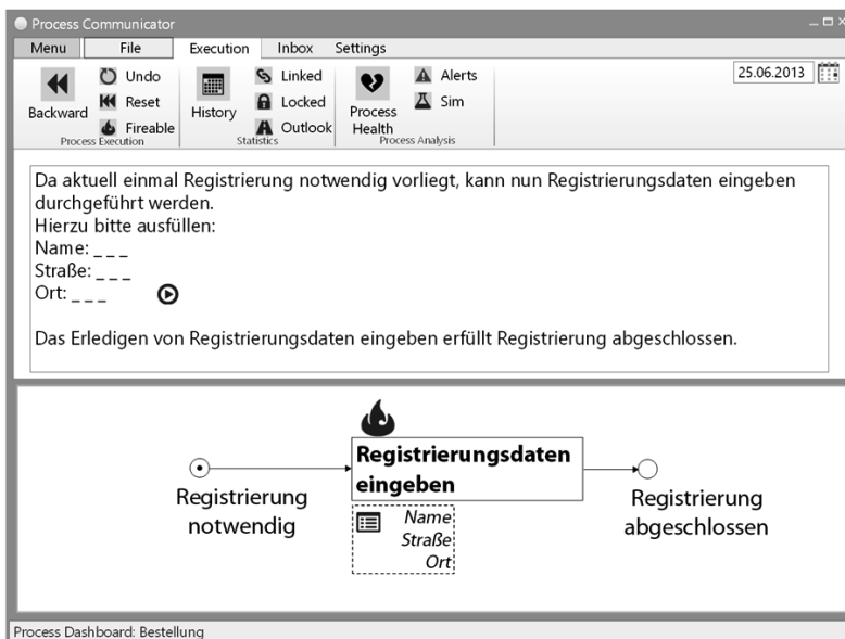
Abb. 6.19: Formulardaten
