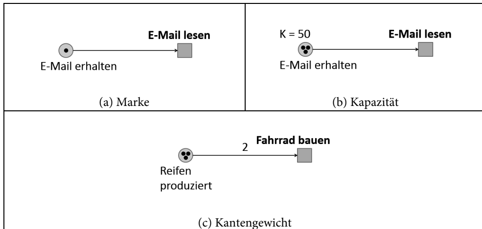
Abb. 5.4: Dynamische Elemente
