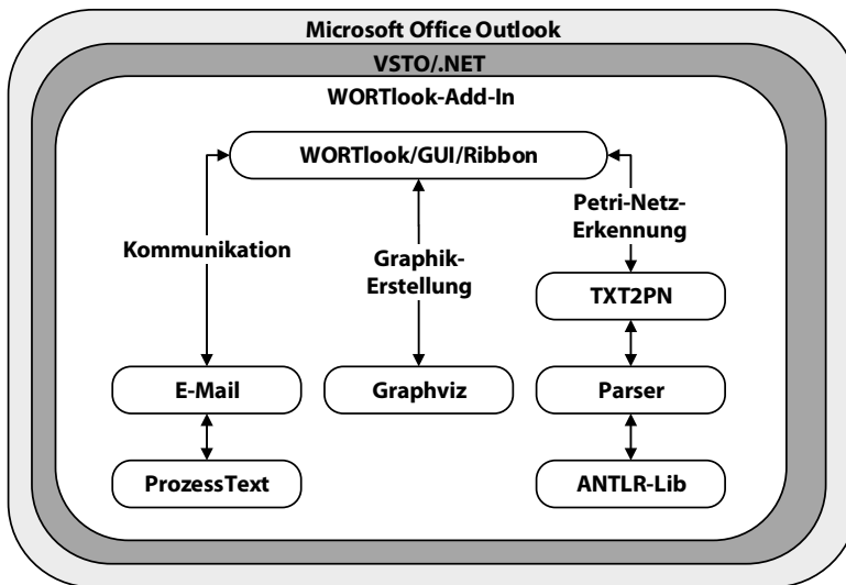
Abb. 6.6: Architektur WORTlook
