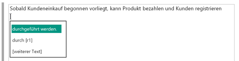
Abb. 6.14: Satz vollenden
