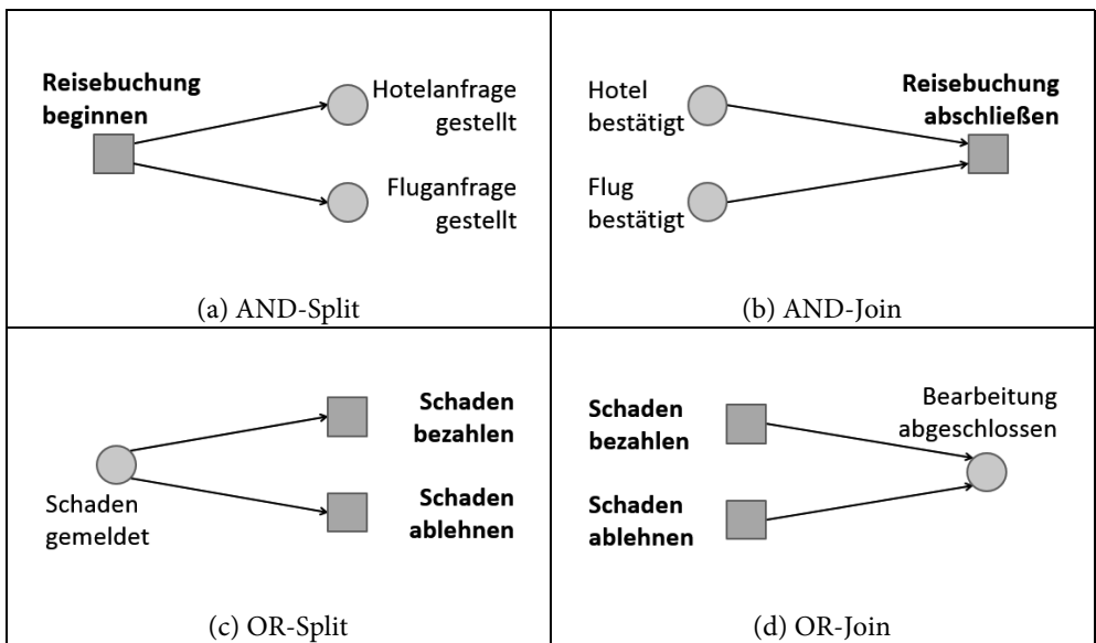
Abb. 5.3: Verzweigungen
