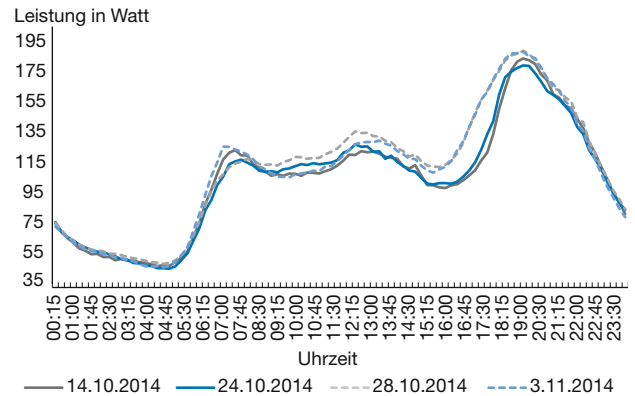
Abbildung 2 Herbst 2014: Tageslastverlauf unmittelbar vor und nach der Zeitumstellung im Netzgebiet Kassel
