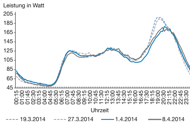
Abbildung 1 Frühjahr 2014: Tageslastverlauf unmittelbar vor und nach der Zeitumstellung im Netzgebiet Kassel
