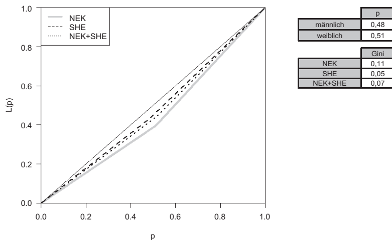
Abbildung 5-11: Lorenzkurve des SHE-Indikators nach Geschlecht
