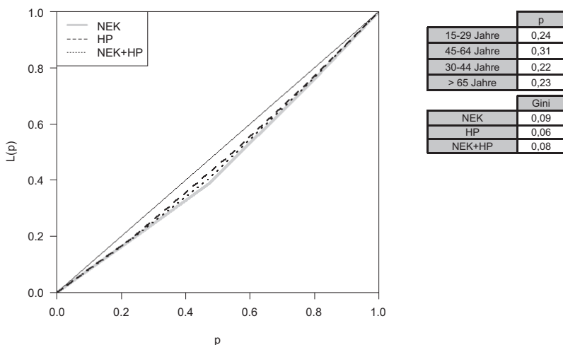
Abbildung 5-6: Lorenzkurve der Teilkomponente Haushaltsproduktion nach Alter
