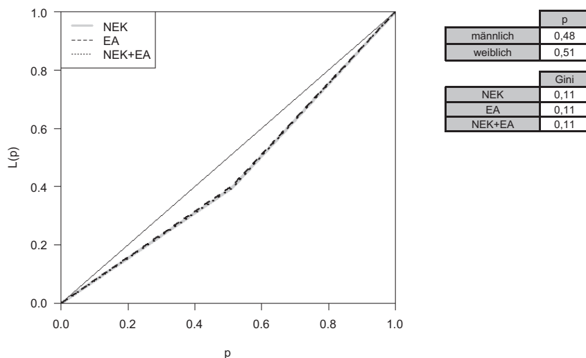
Abbildung 5-8: Lorenzkurve der Teilkomponente Ehrenamt nach Geschlecht
