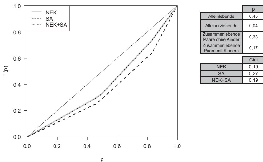
Abbildung 5-4: Lorenzkurve der Teilkomponente Schwarzarbeit nach Haushaltstyp
