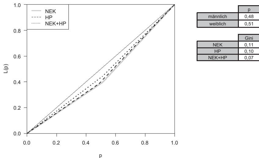
Abbildung 5-5: Lorenzkurve der Teilkomponente Haushaltsproduktion nach Geschlecht
