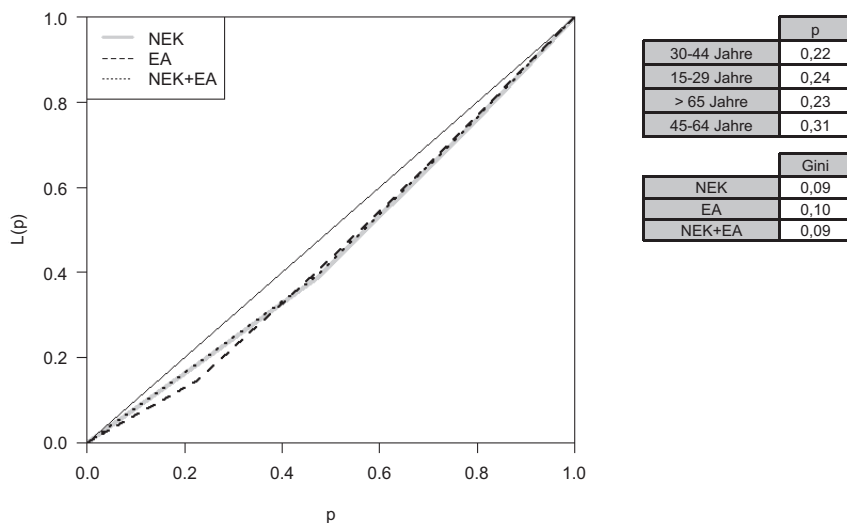
Abbildung 5-9: Lorenzkurve der Teilkomponente Ehrenamt nach Alter
