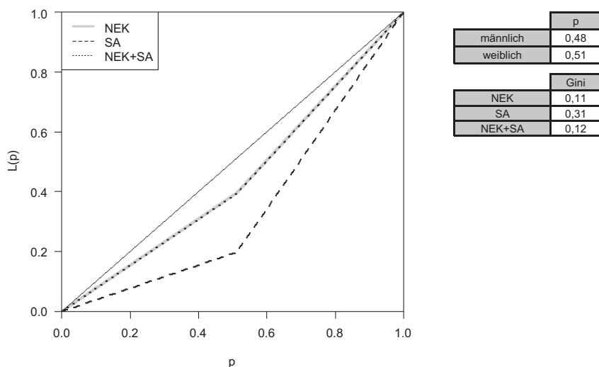
Abbildung 5-2: Lorenzkurve der Teilkomponente Schwarzarbeit nach Geschlecht
