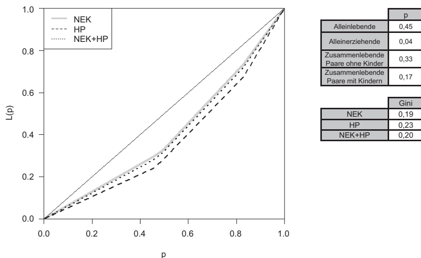
Abbildung 5-7: Lorenzkurve der Teilkomponente Haushaltsproduktion nach Haushaltstyp
