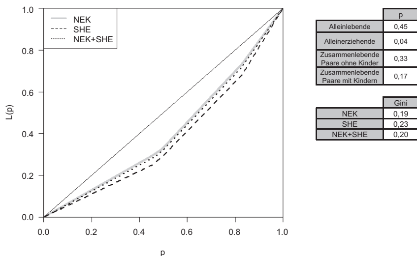
Abbildung 5-13: Lorenzkurve des SHE-Indikators nach Haushaltstyp
