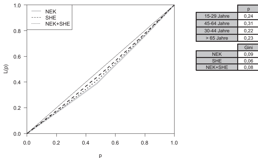
Abbildung 5-12: Lorenzkurve des SHE-Indikators nach Alter
