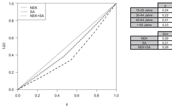
Abbildung 5-3: Lorenzkurve der Teilkomponente Schwarzarbeit nach Alter
