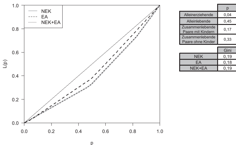
Abbildung 5-10: Lorenzkurve der Teilkomponente Ehrenamt nach Haushaltstyp
