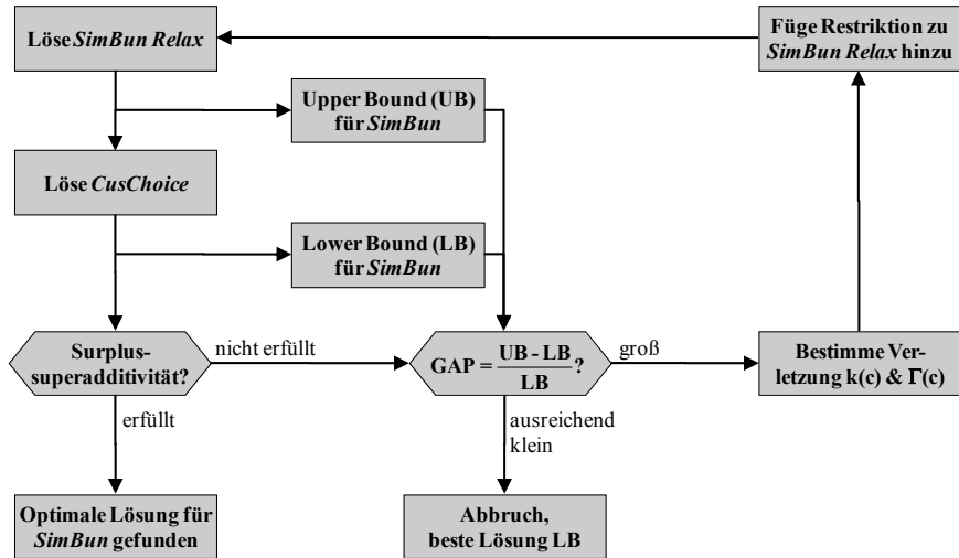
Abbildung 4.4: Ablauf der Produktprogrammoptimierung mit simultaner Preisbündelung
