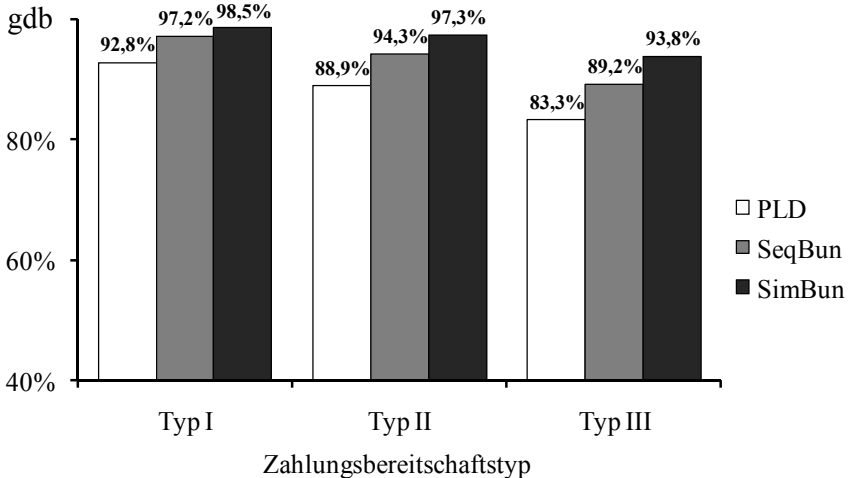
Abbildung 5.22: Anteil des Gesamtdeckungsbeitrags an der maximal möglichen Wohlfahrt in Abhängigkeit des Zahlungsbereitschaftstyps für segmentvieler Varianten
