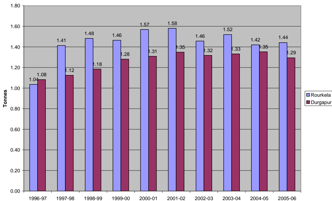
Sinter Use Per tonne of Hot Metal
