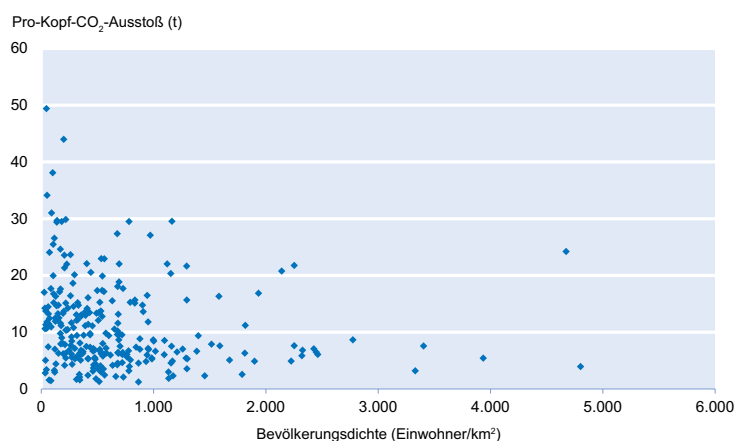
Abb. 1 Pro-Kopf-CO 2 -Ausstoß abhängig von der Bevölkerungsdichte
